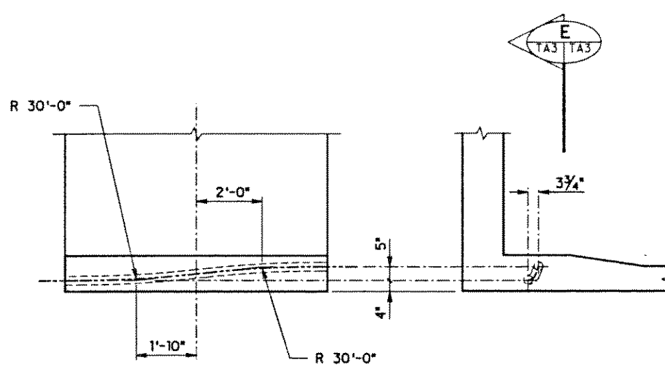
SECTION SCALE: 1/2" = 1'-0"
