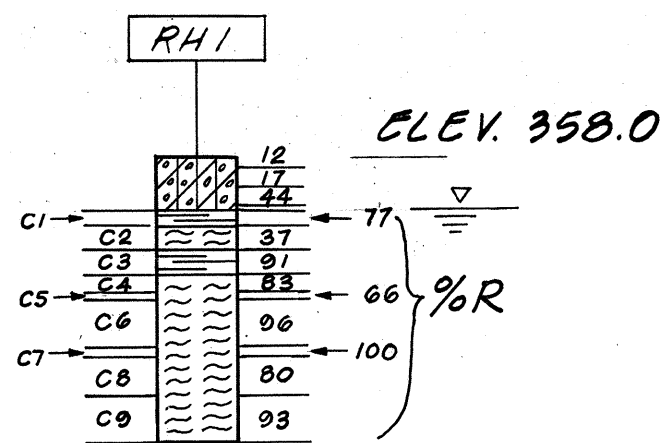
BORING RH1
