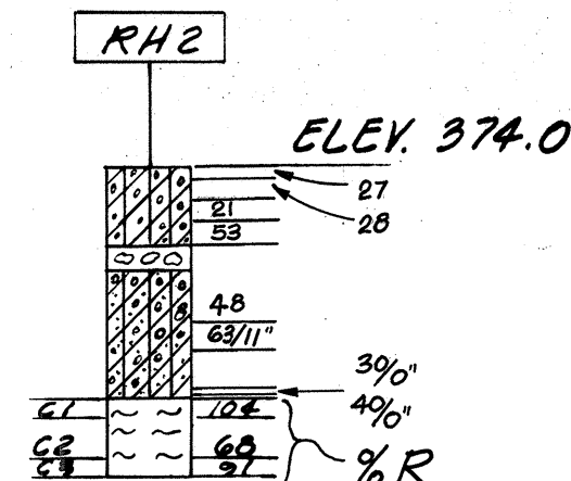
BORING RH2
