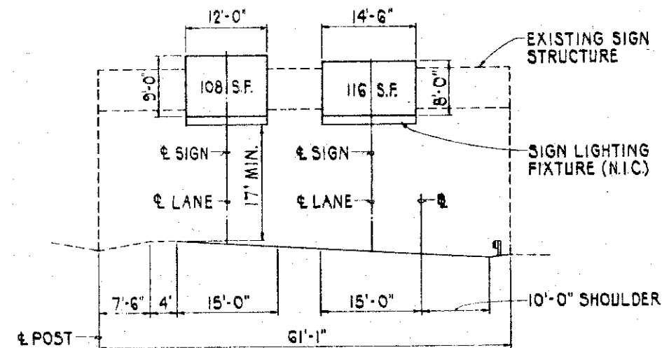
SIGN E-4 RAMP N @ STA. 34 + 87 SCALE: 1"=10'
