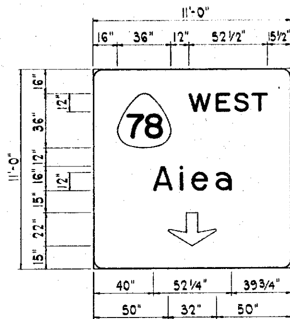
SIGN E-2L SCALE: 3/8" = 1'-0"
