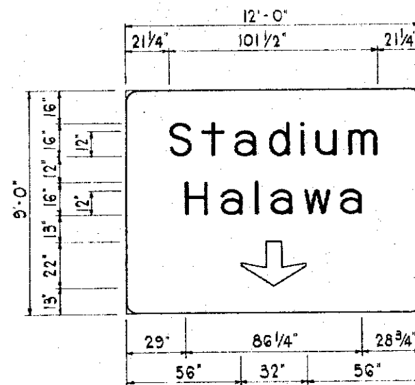
SIGN E-4L SCALE: 3/8"=1'-0"
