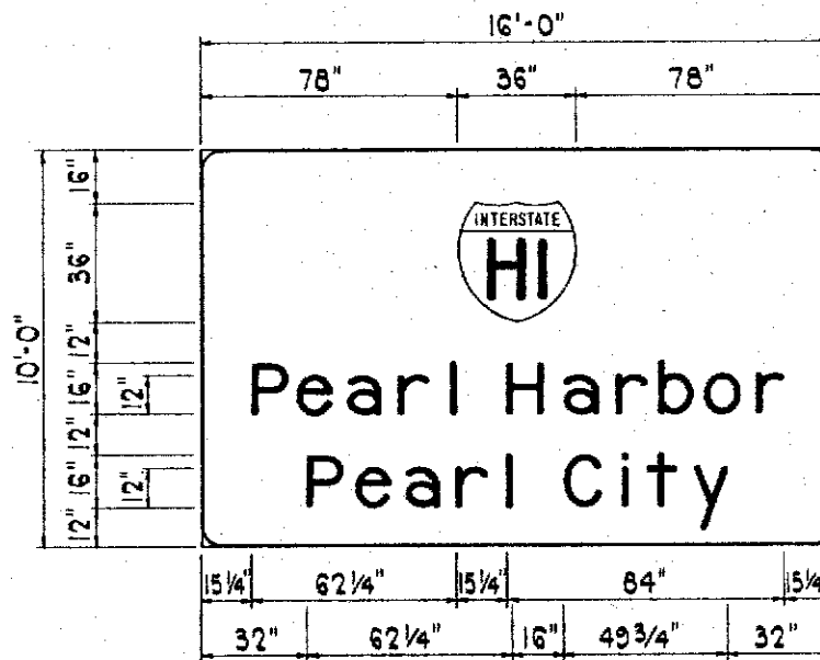
SIGN E-3L SCALE: 3/8" = 1'-0"
