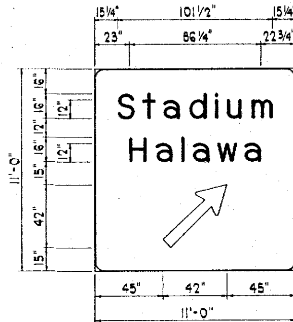
SIGN E-2R SCALE: 3/8" = 1'-0"
