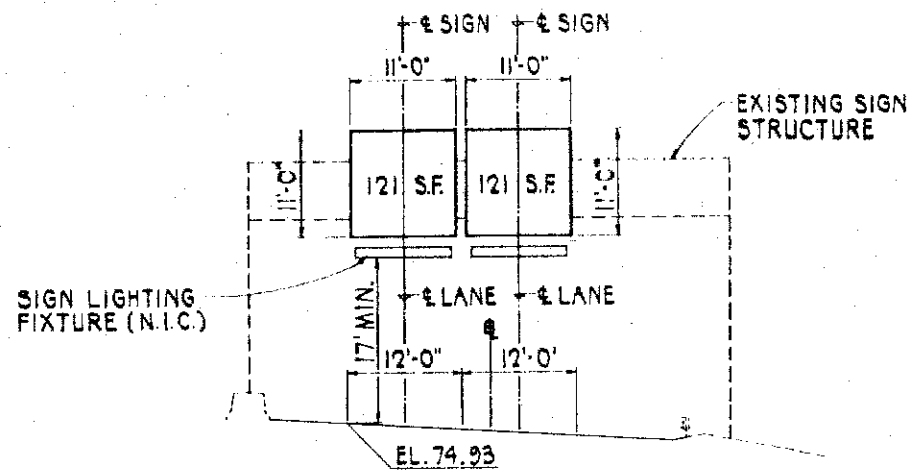
SIGN E-2 RAMP M @ STA. 19 + 33 SCALE: 1"=10'
