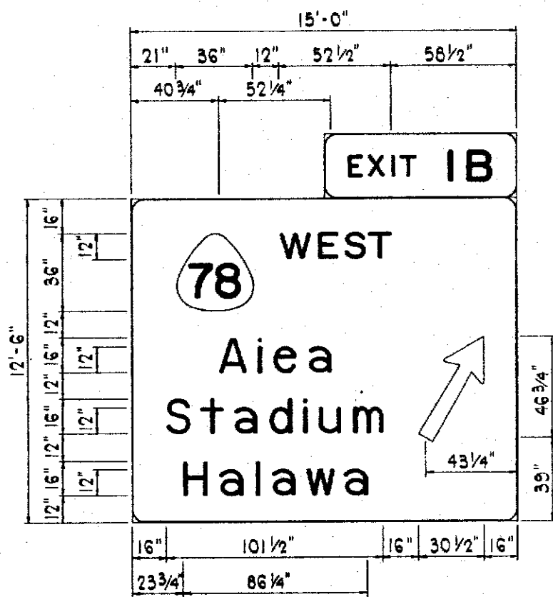
SIGN E-1 SCALE: 3/8" = 1'-0"
