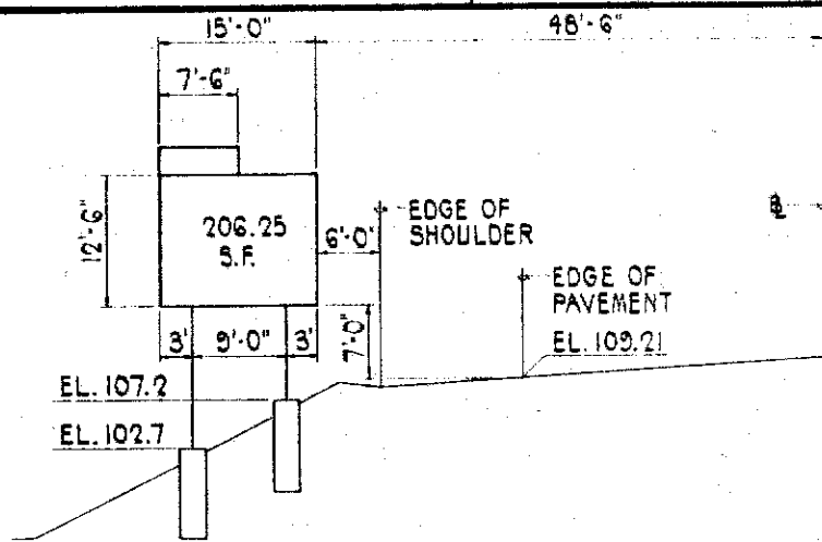
SIGN E-1 H-3 @ STA. 345 + 00 SCALE: 1"=10'
