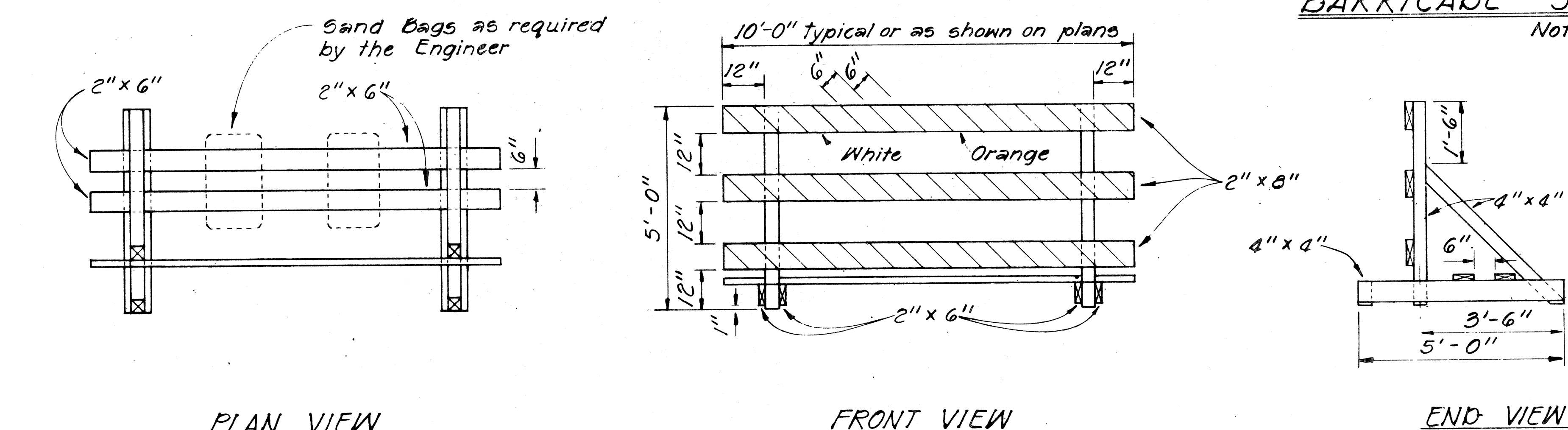
TYPE III BARRICADE Scale: 1/2" = 1'-0"
