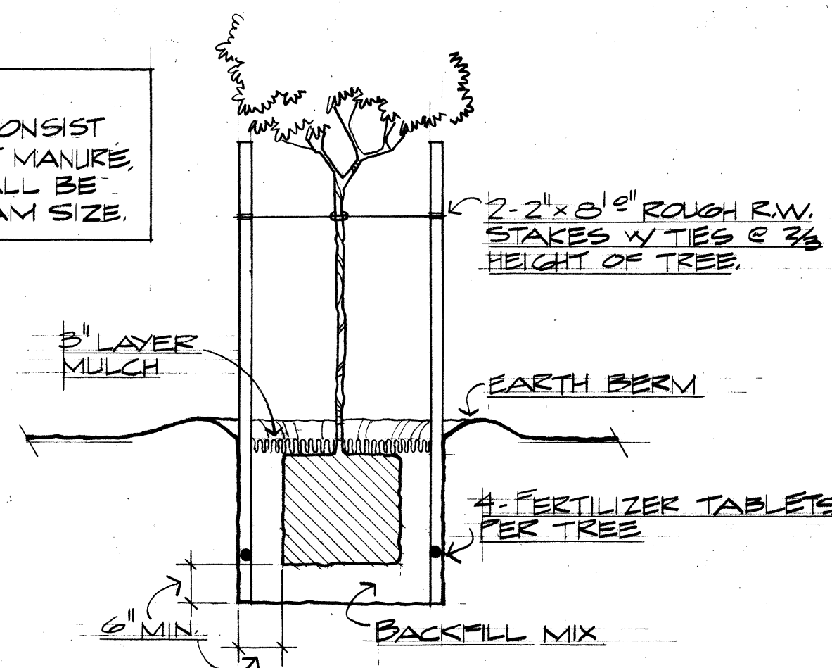
TYP. 5 G.C. TREE PLANTING DET. NO SCALE
