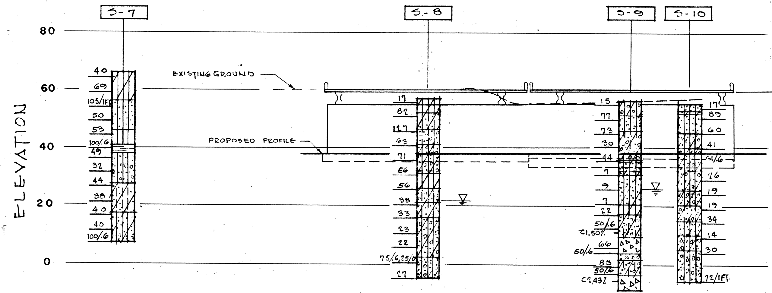
SECTION A-A
