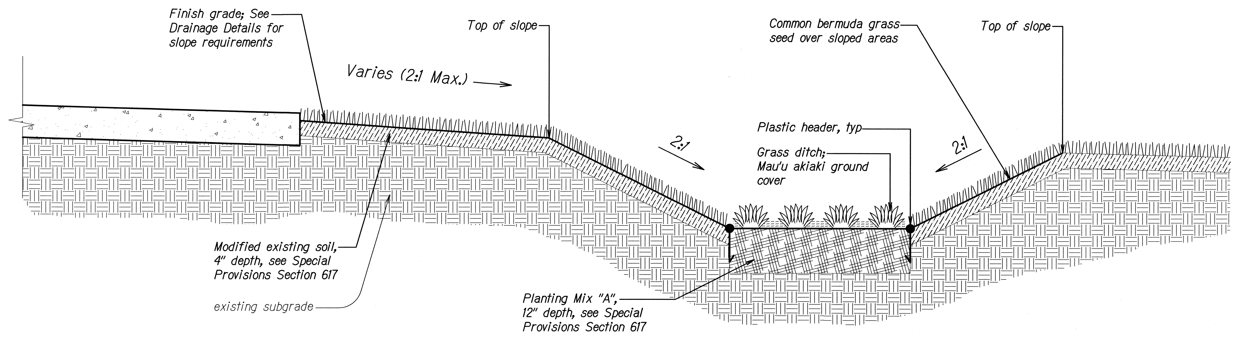
3 SECTION THRU GRASS DITCH Scale: 1" = 1'-0"
