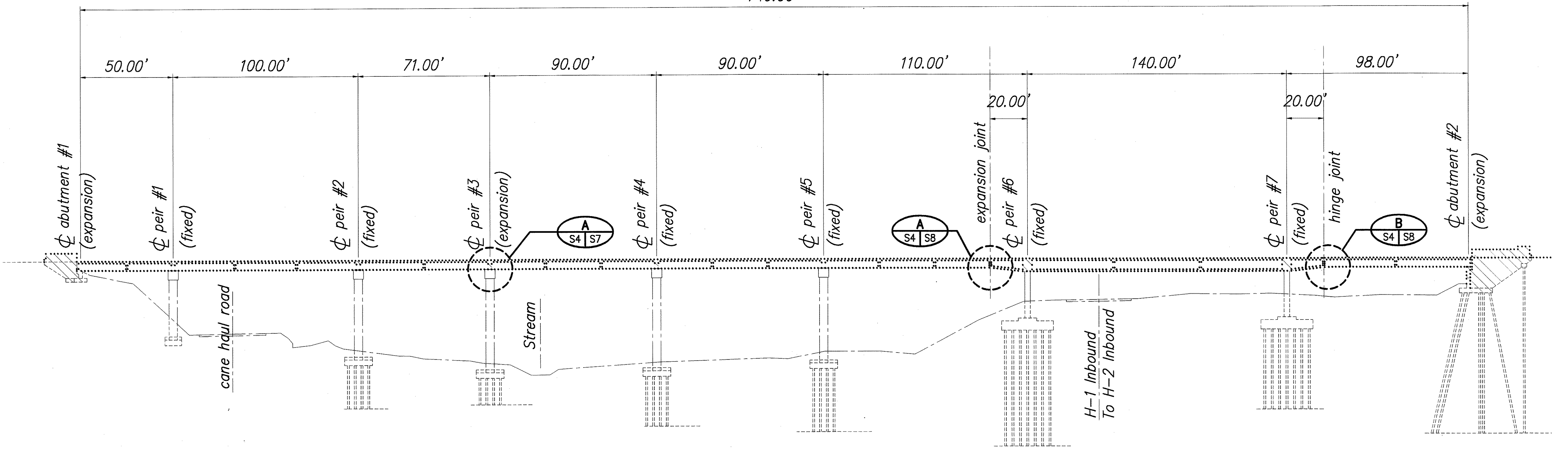
LONGITUDINAL SECTION – STRUCTURE 15 SCALE: 1" = 30'
