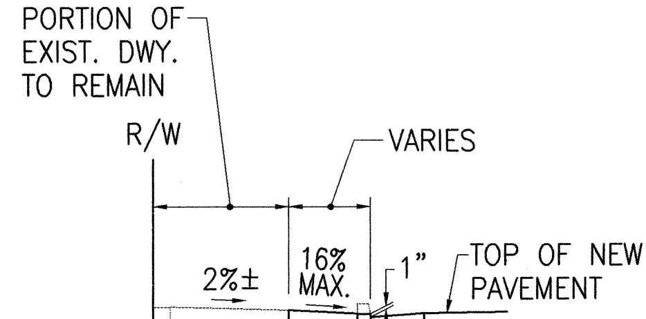
DETAIL DG SCALE: 1"=10'
