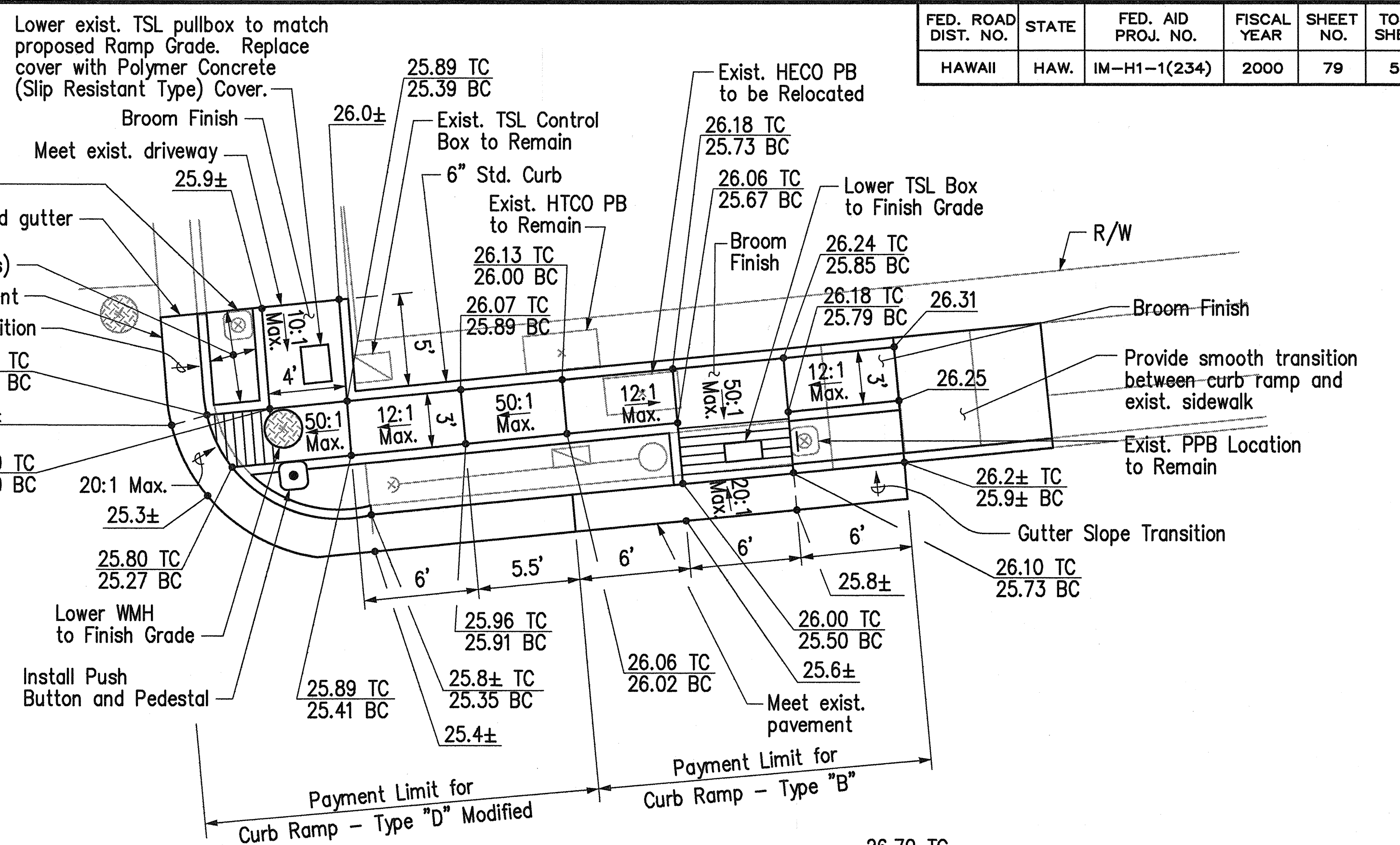
DETAIL A Scale: 1" = 5'
