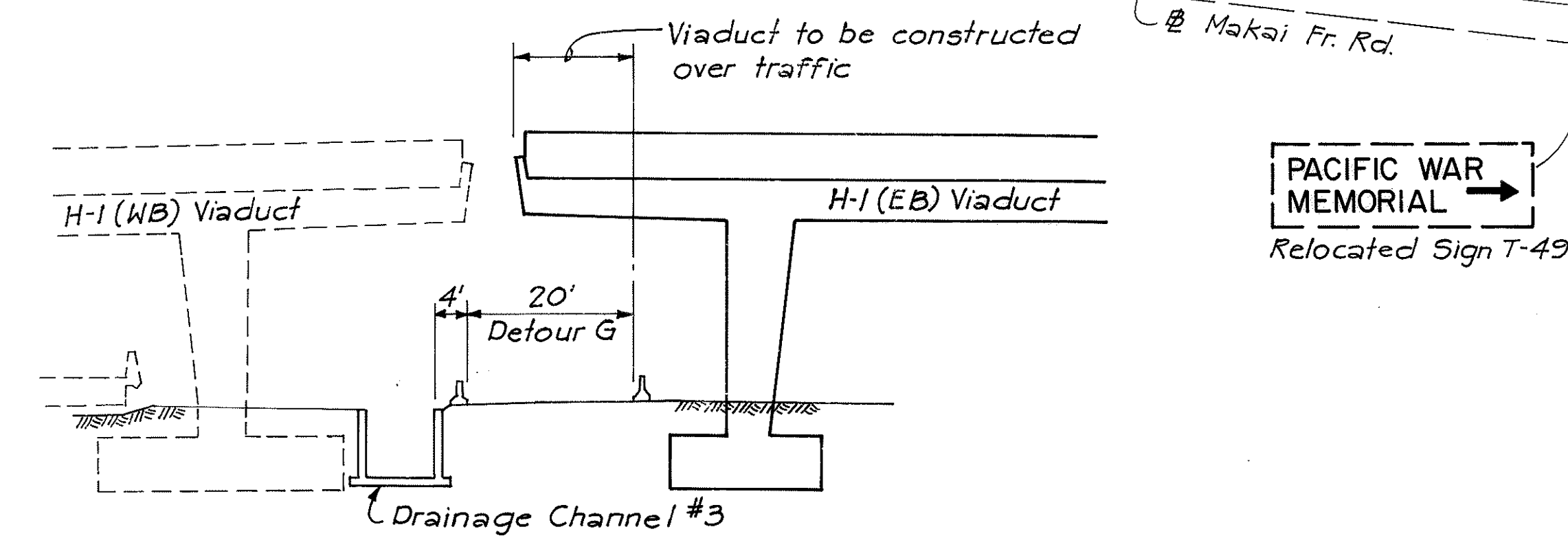
SECTION A N.T.S. P-2/P-2
