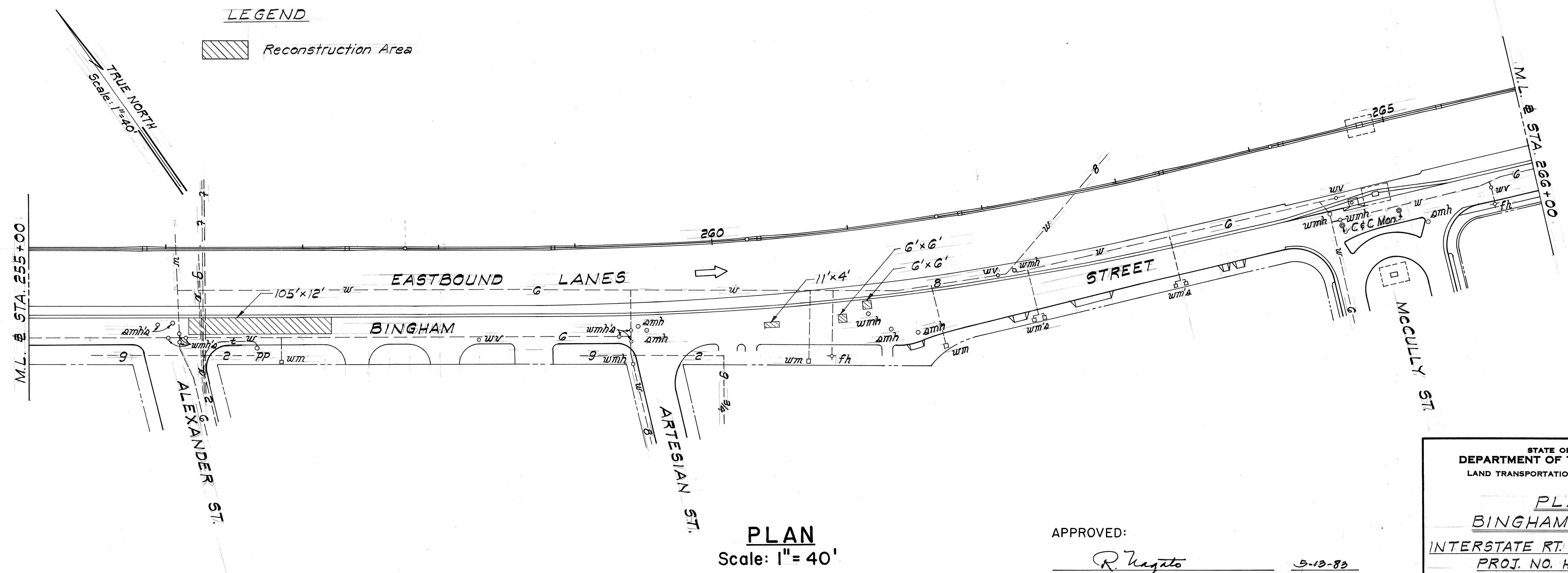
PLAN Scale: 1"=40'
