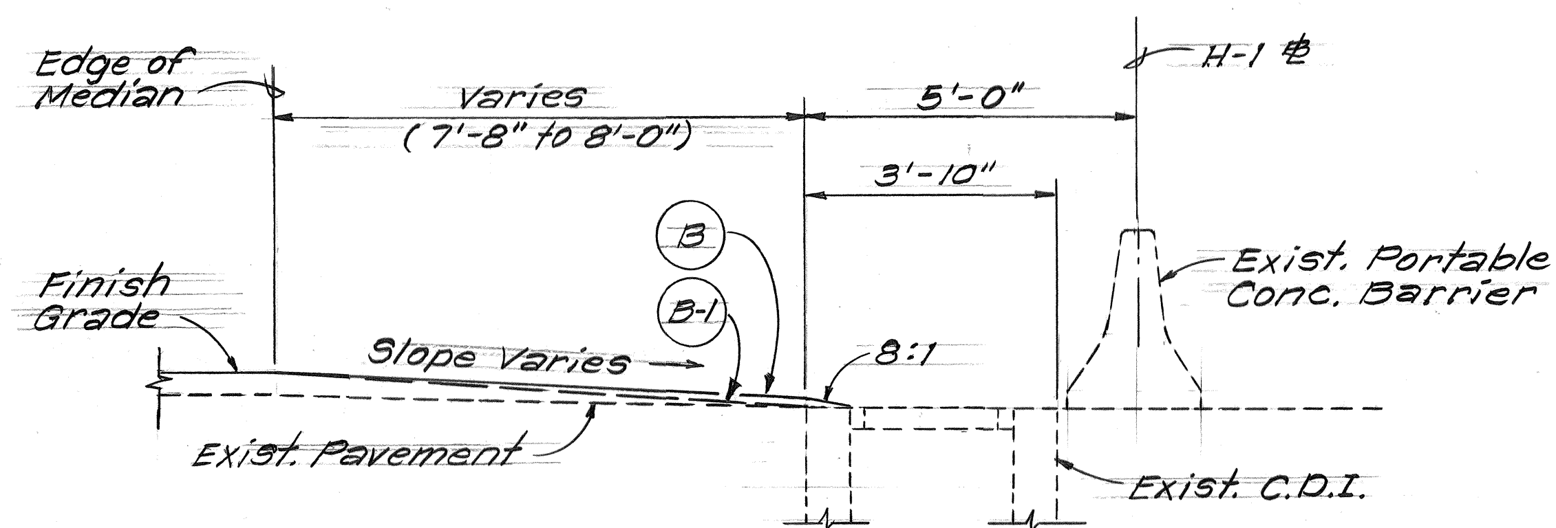
SECTION B (C.D.I. @ STA. 39+00, 43+00 & 44+00 ONLY) SECTION B-1 (C.D.I. @ STA. 40+00, 41+00, 42+00 & 45+00) Scale: 1/2" = 1'-0"
