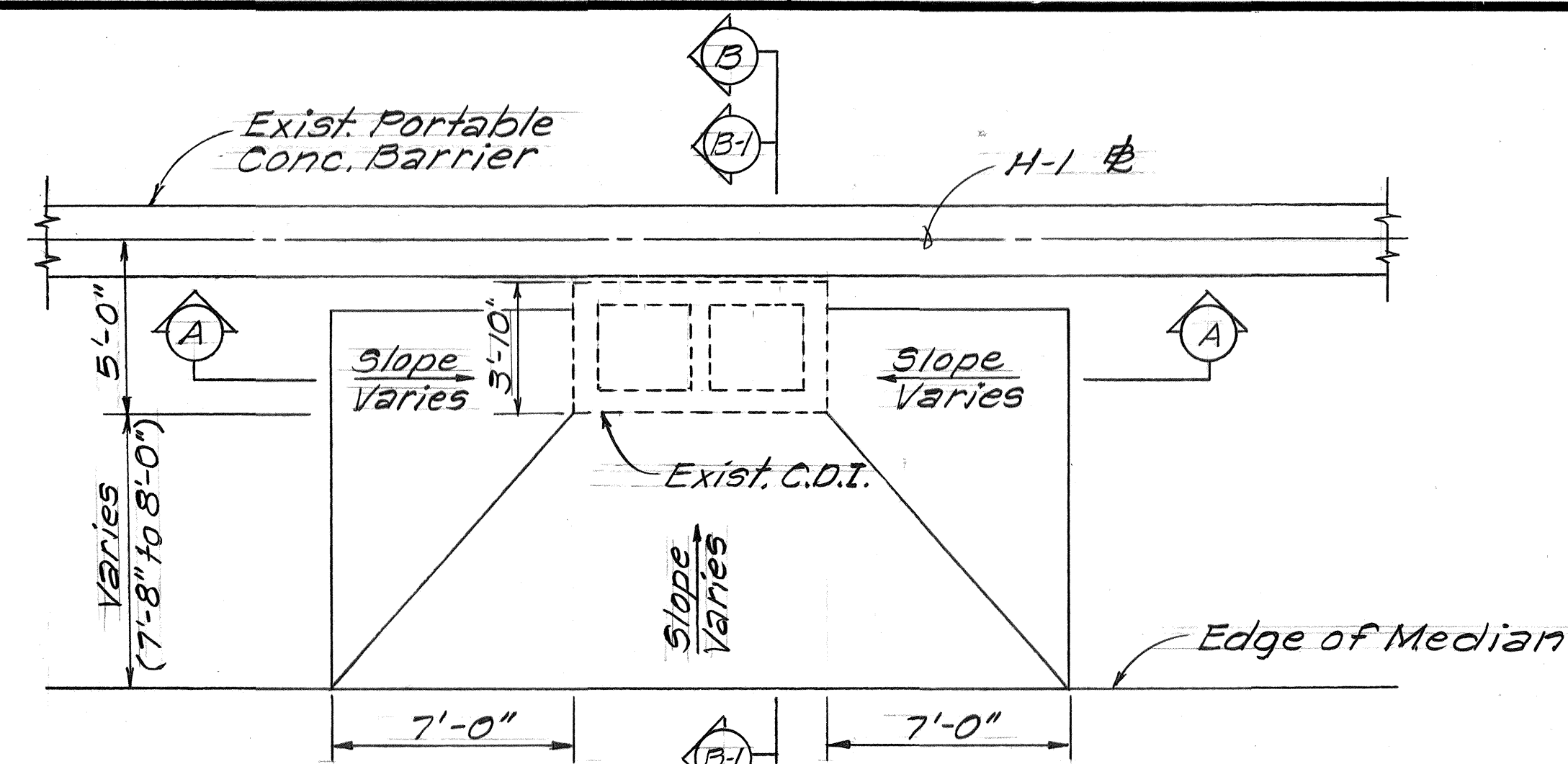
PLAN Scale: 1/4" = 1'-0"
