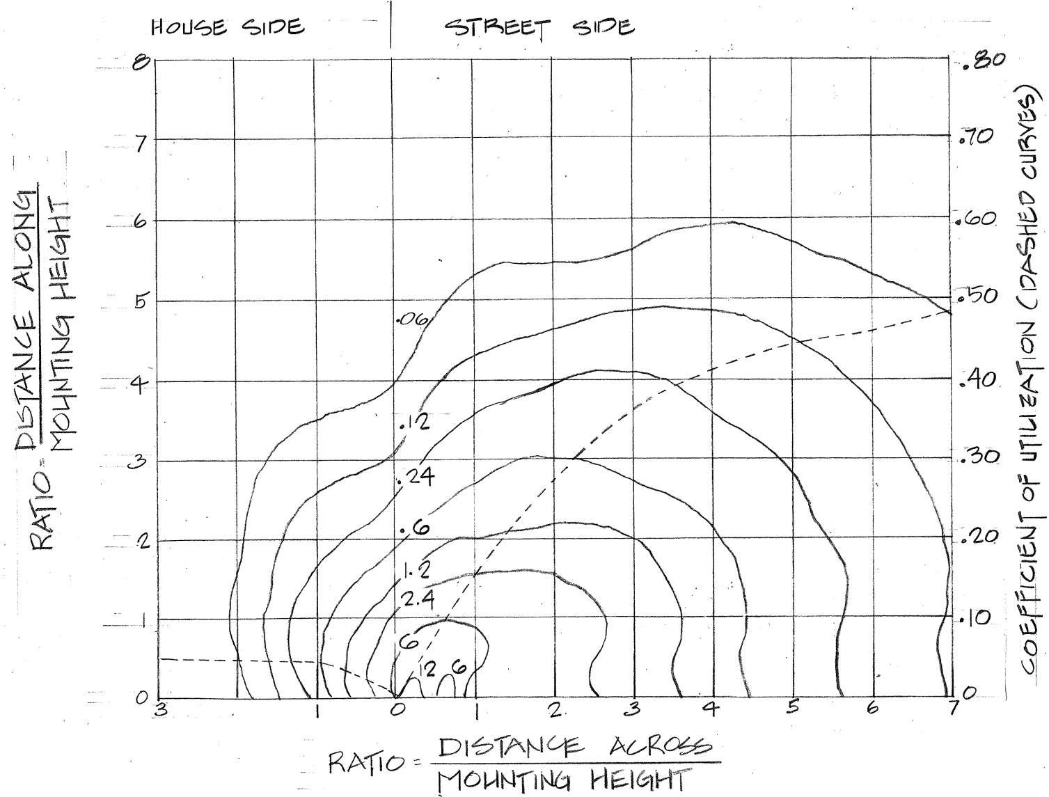
ISOFOOTCANDLE DIAGRAM
