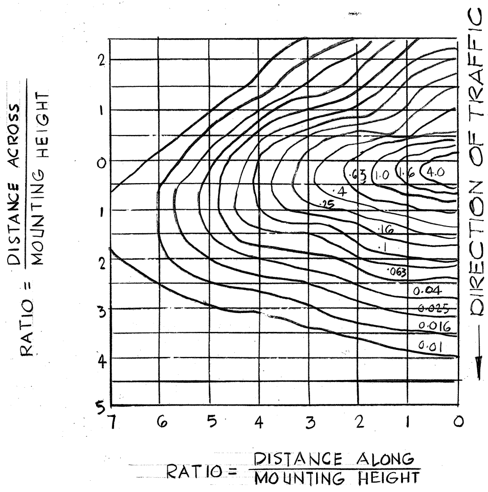
ISOFOOTCANDLE DIAGRAM
