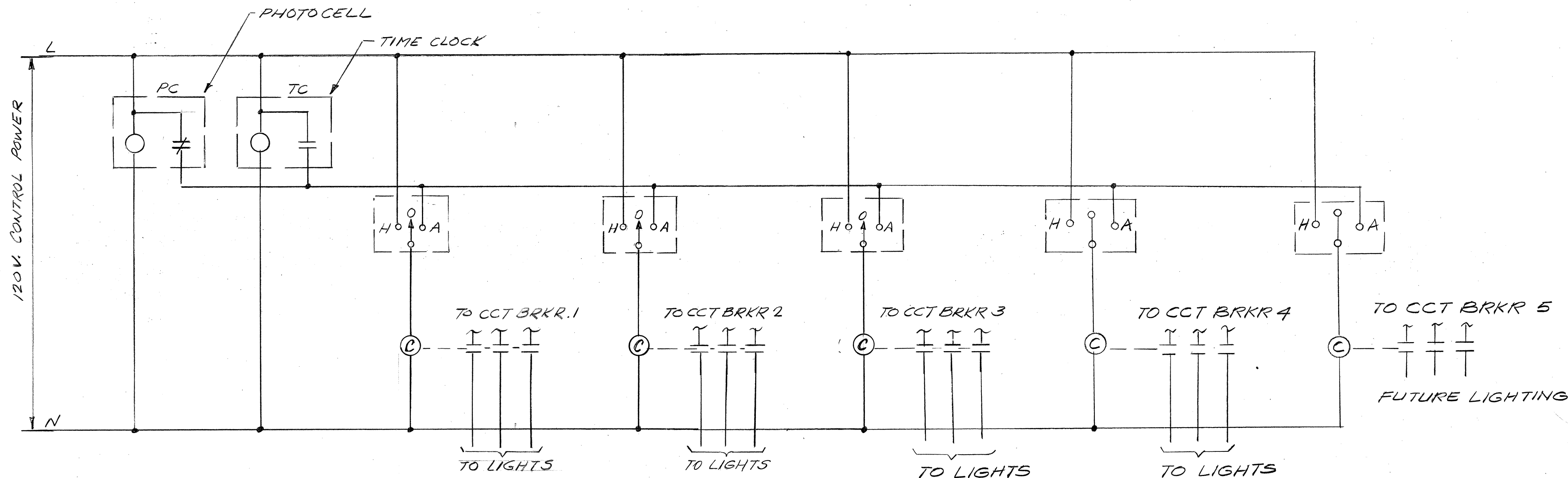
CONTROL SCHEMATIC N.T.S.
