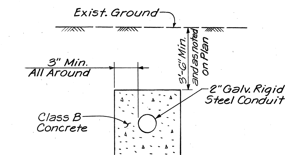
CONDUIT CONCRETE ENCASEMENT N.T.S.
