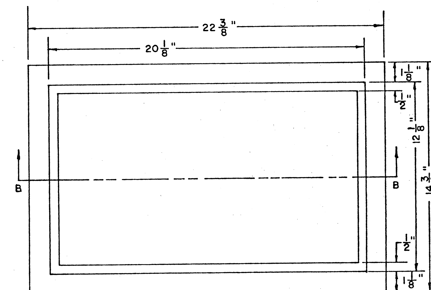
TOP VIEW OF FRAME N.T.S.
