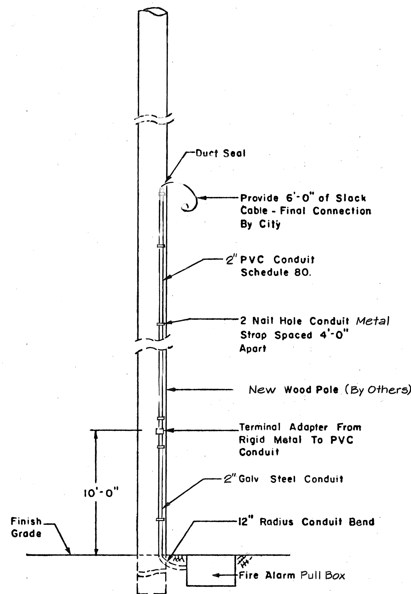
FIRE ALARM CONDUIT RISER DETAIL (JP-1) N.T.S.
