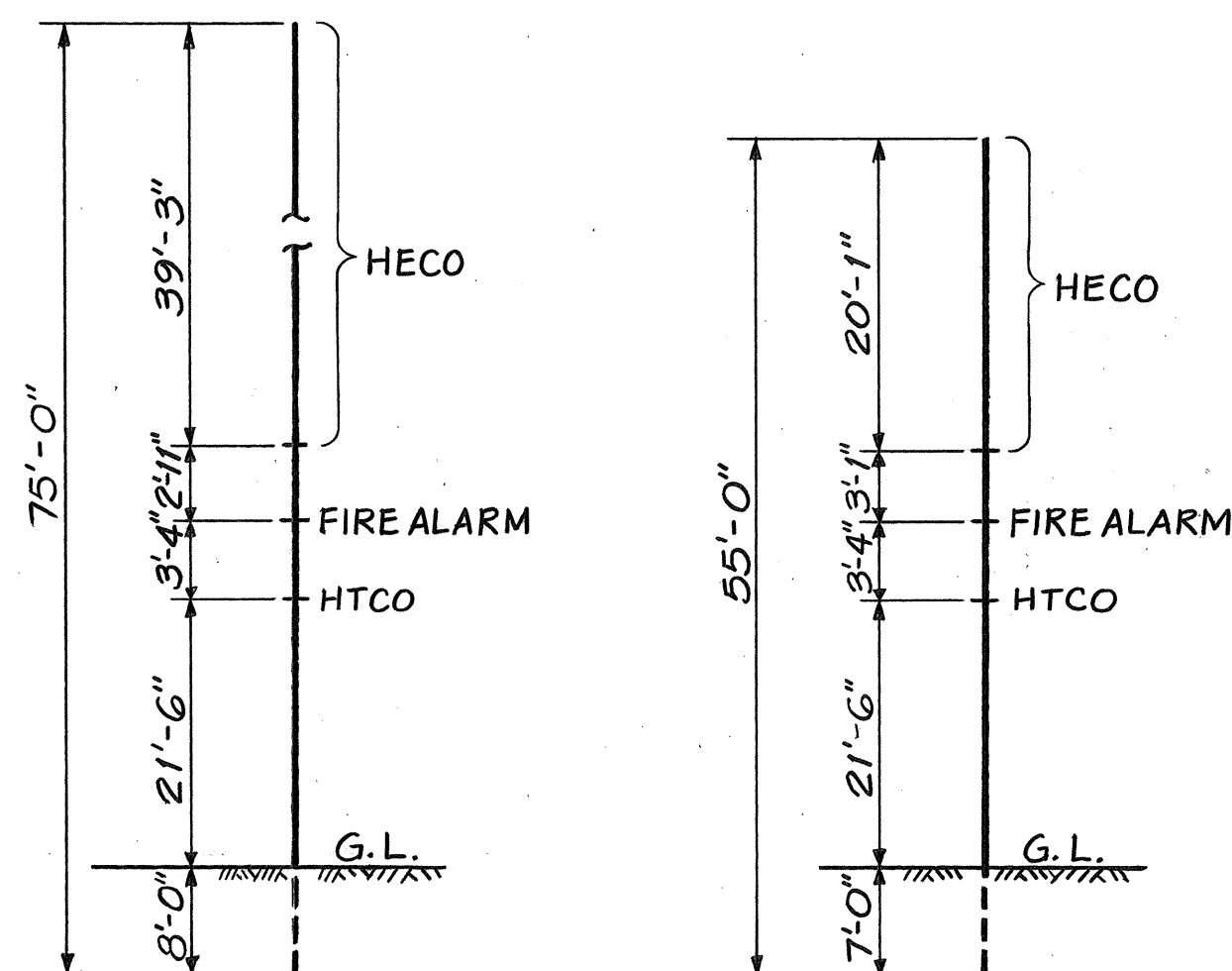
JP-1, 75' POLE AT PUULOA ROAD N.T.S.
