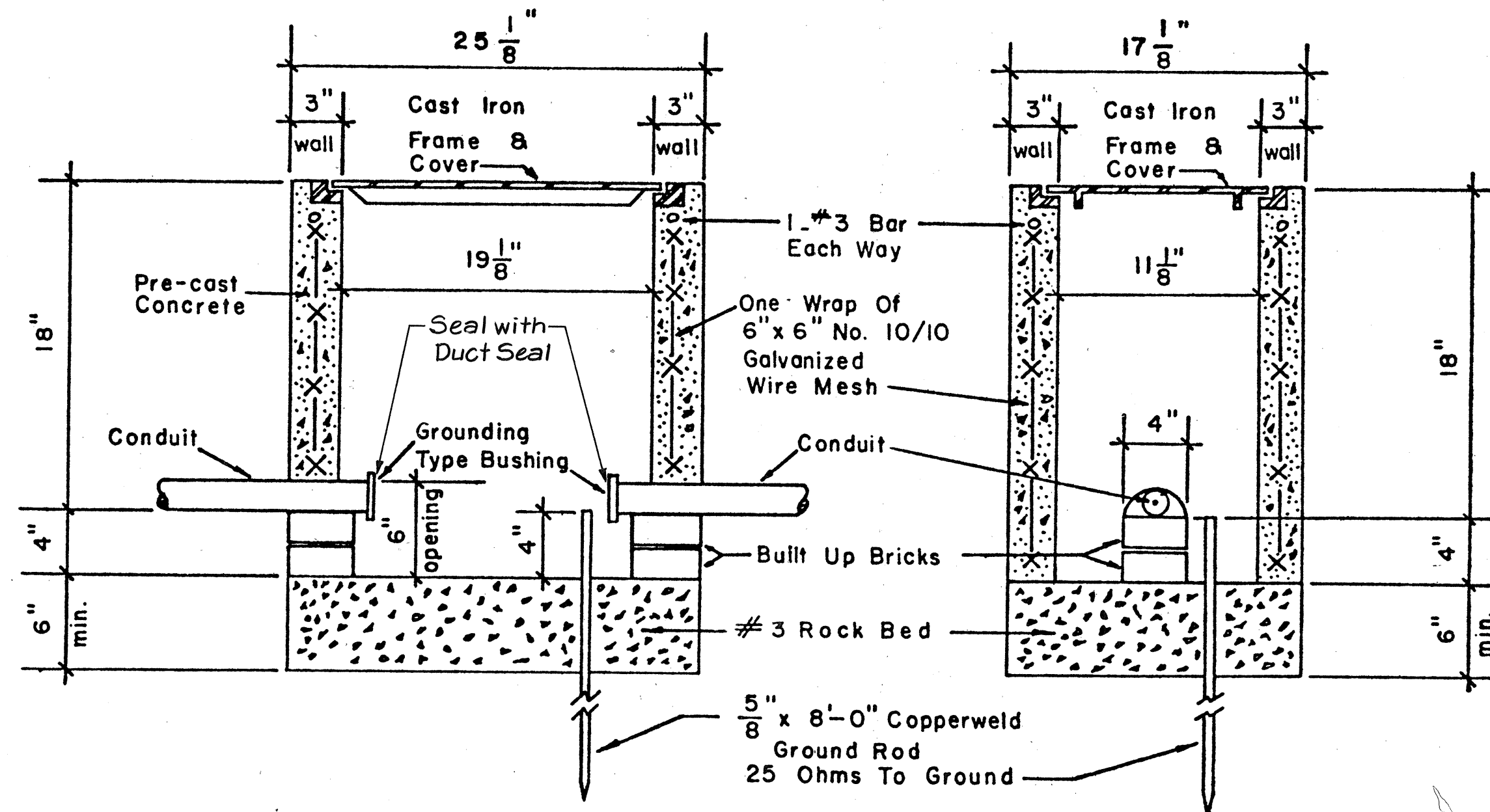
PRECAST PULLBOX N.T.S.
