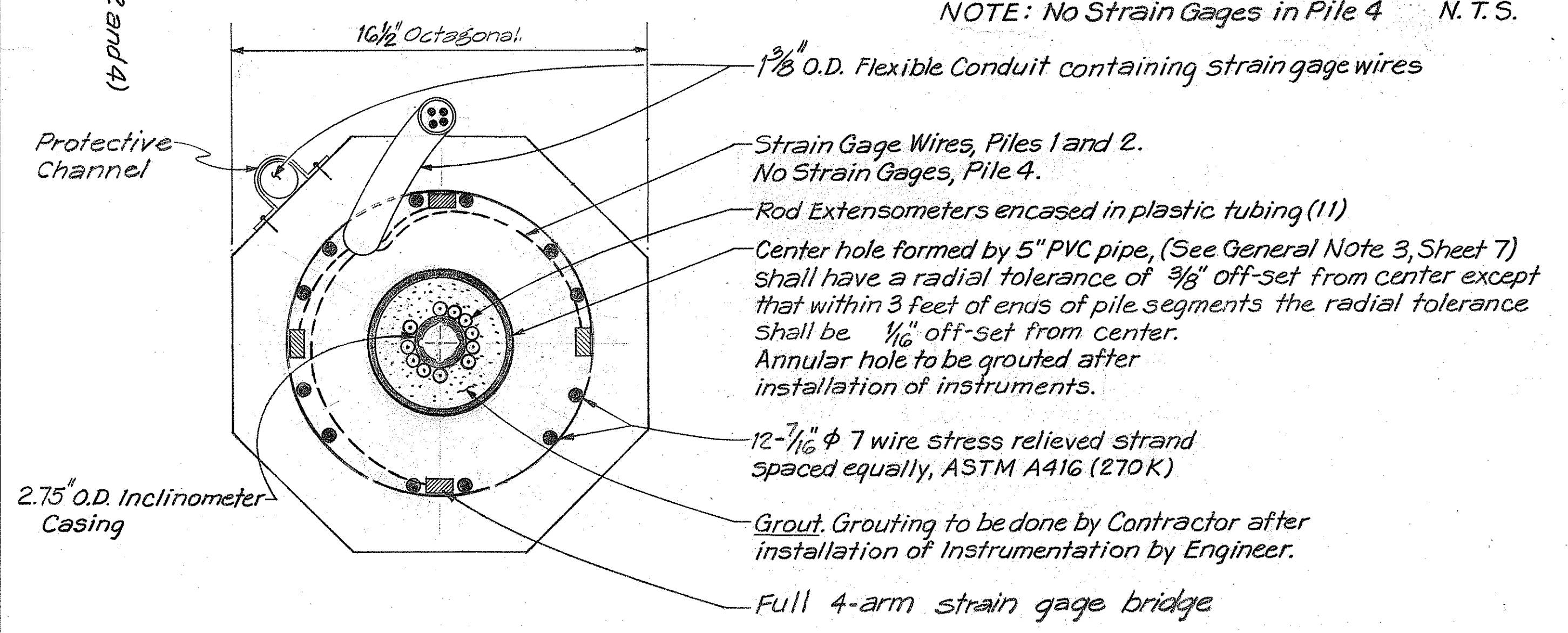
SECTION A-A Scale: 3"=1'-0"
