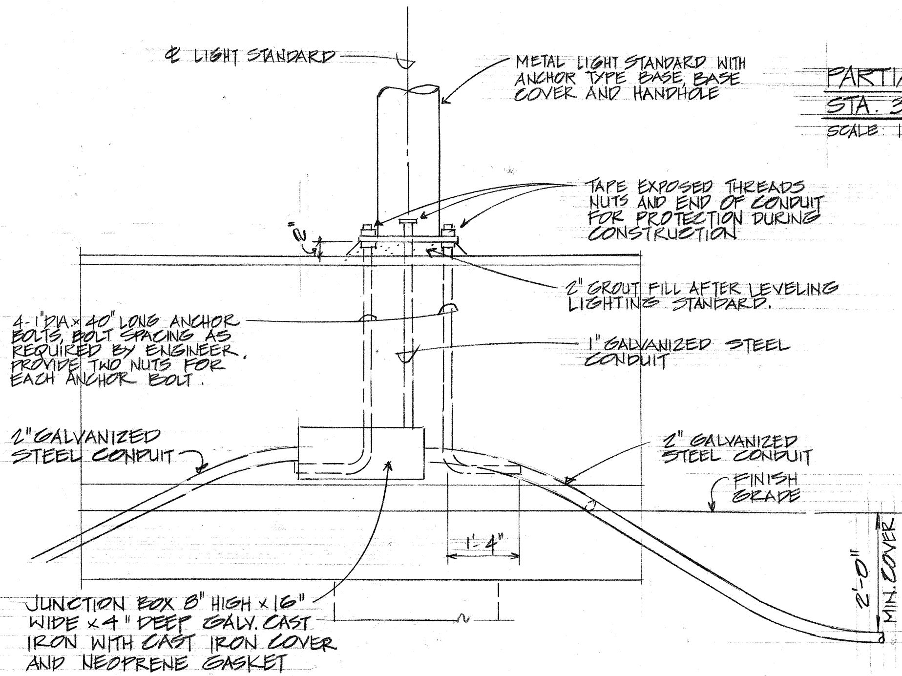
1.1 ELEVATION E-2 SCALE: 1"=1'-0"
