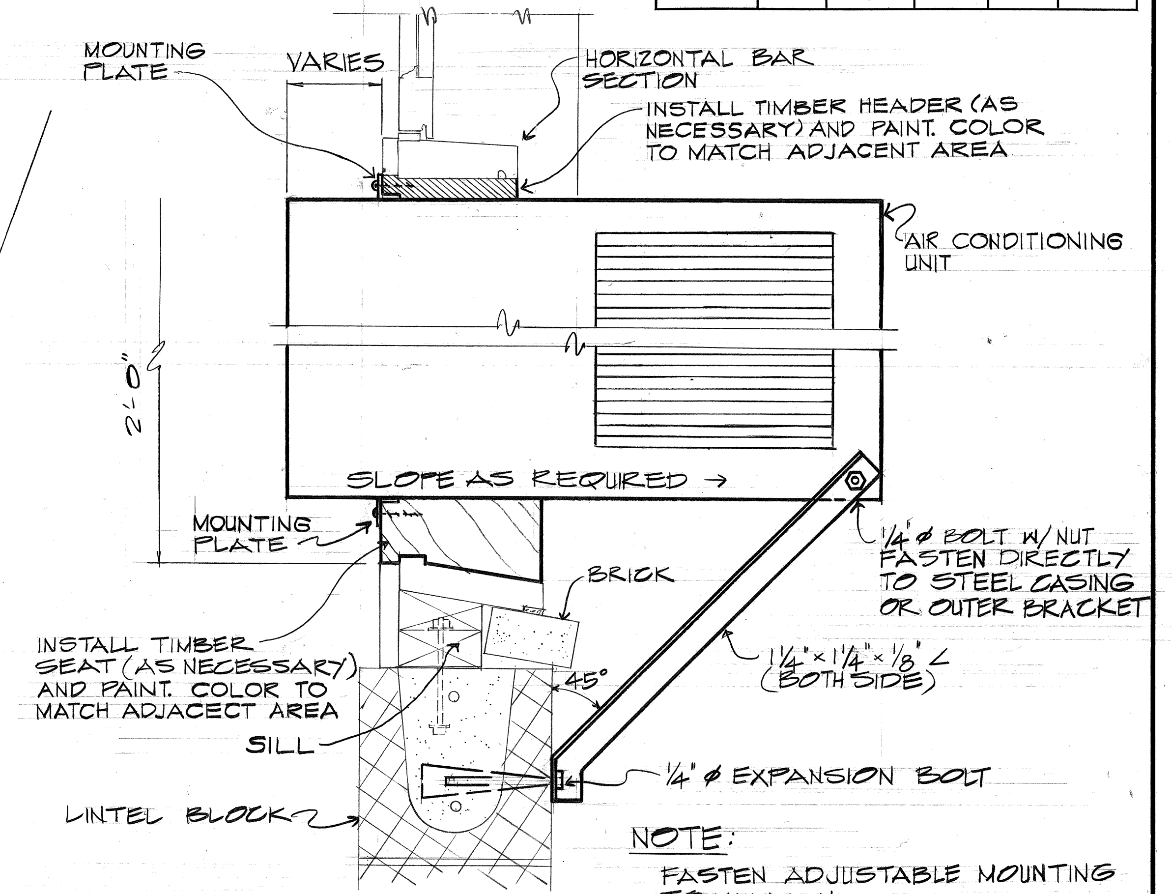
SECTION SCALE: 3"=1'-0"
