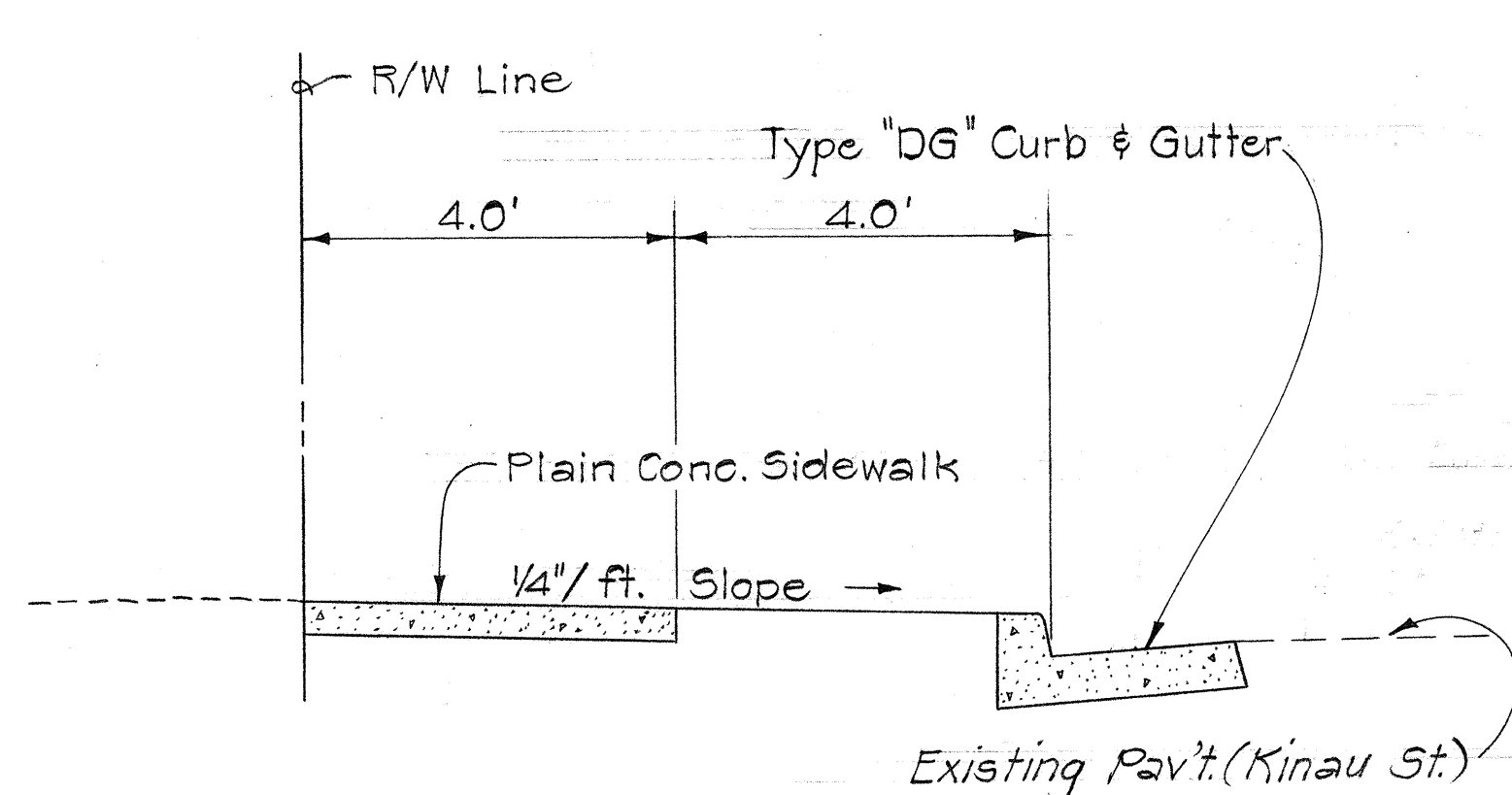
SECTION "A-A" Scale: 1/2" = 1'-0"
