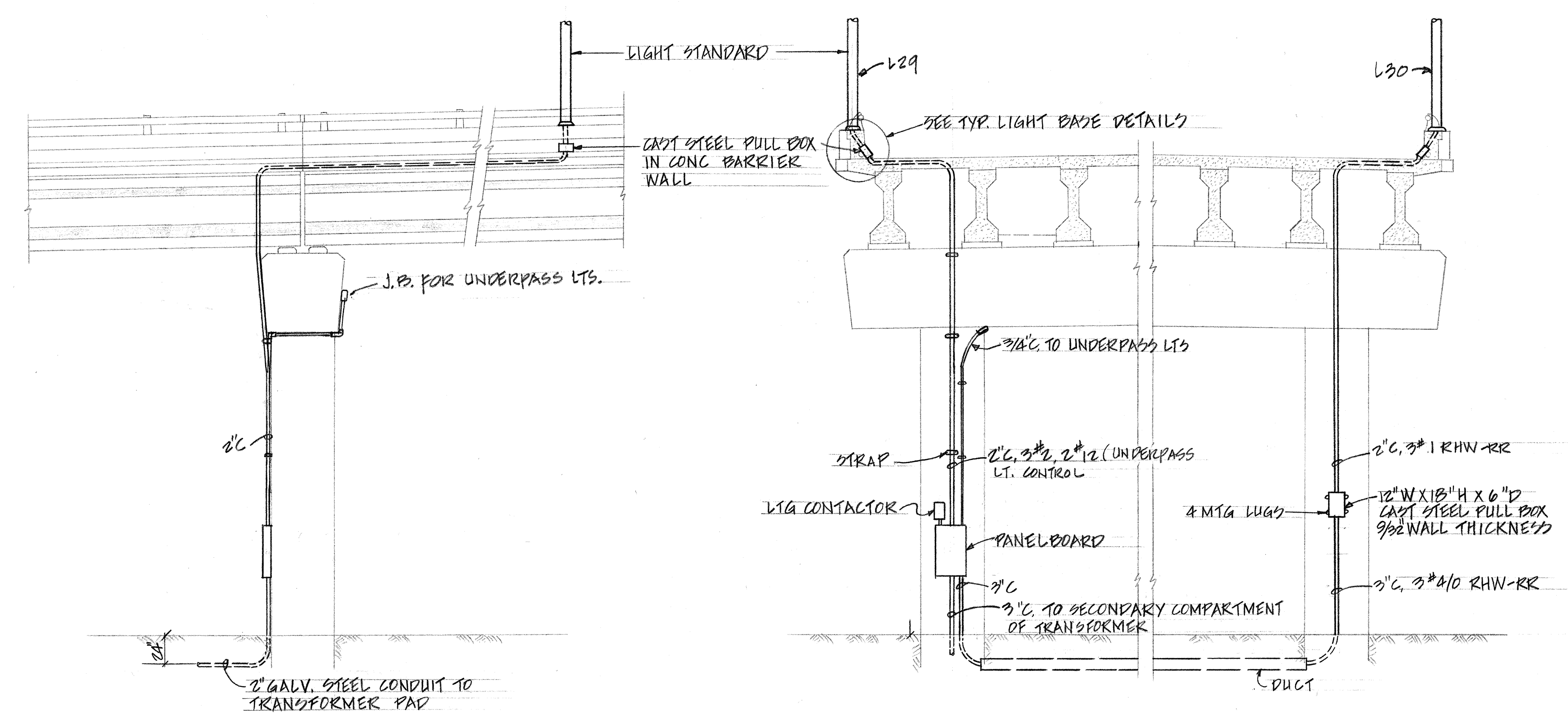
SECTION A SCALE: 3/16" = 1'-0"
