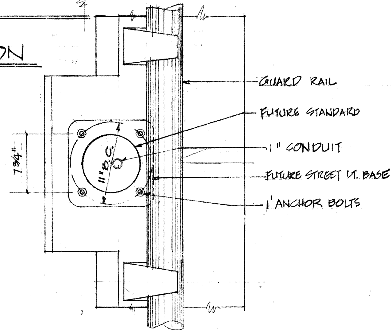
PLAN SCALE: 1 1/2" = 1'-0"
