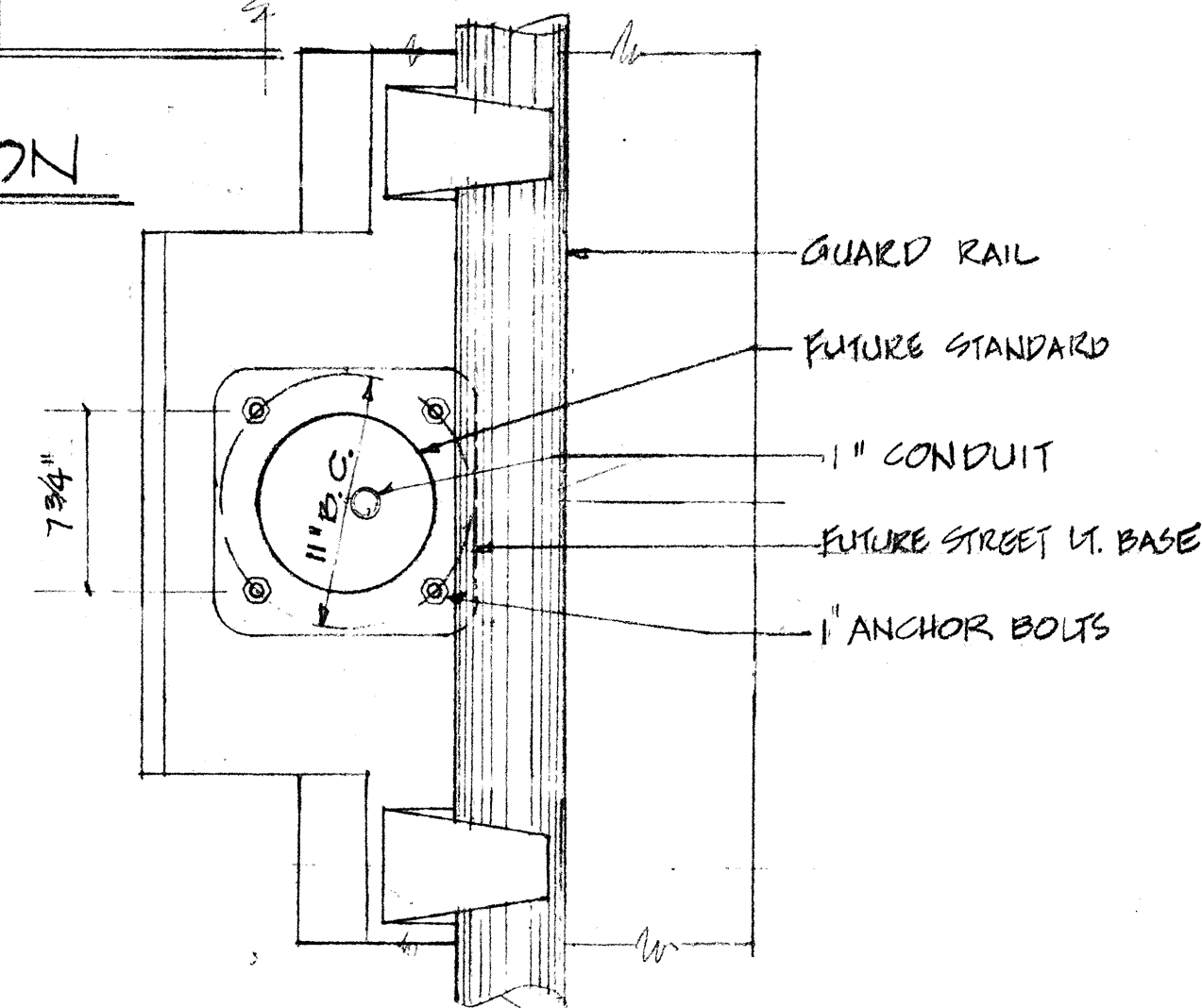
PLAN SCALE: 1 1/2" = 1'-0"
