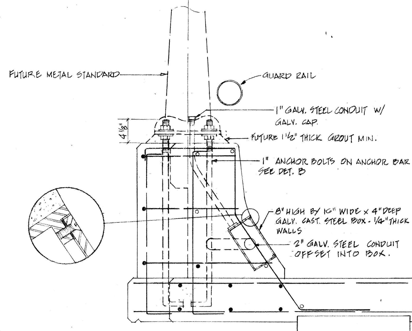
SECTION SCALE: 1 1/2" = 1'-0"
