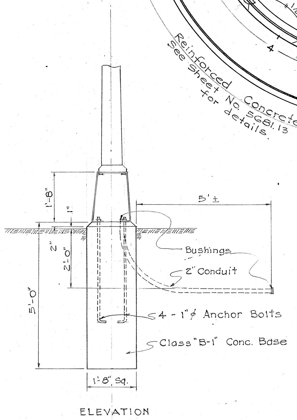
ELEVATION
