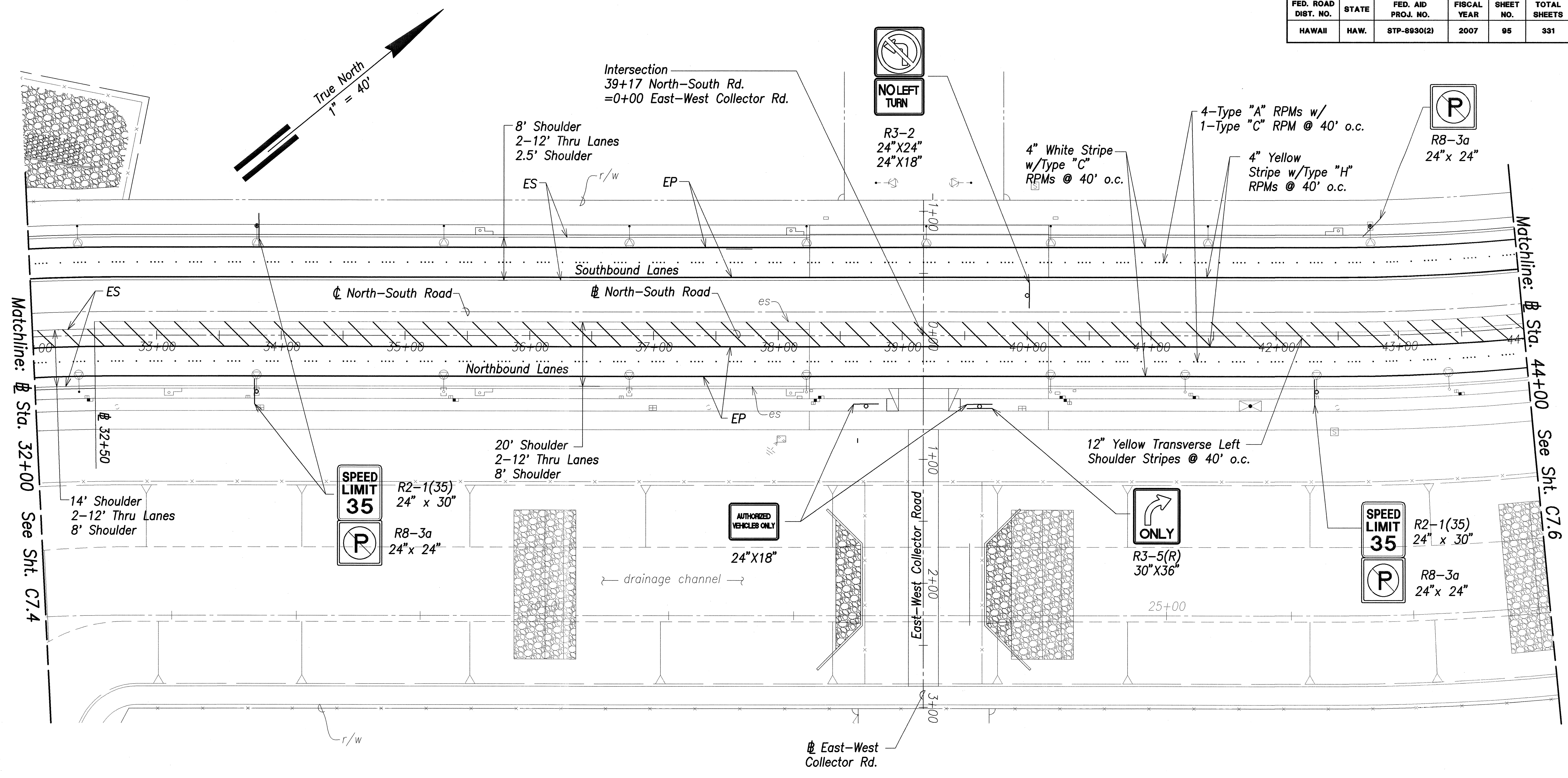
Striping Plan - Sta. 32+00 to Sta. 44+00 Scale: 1" = 40'
