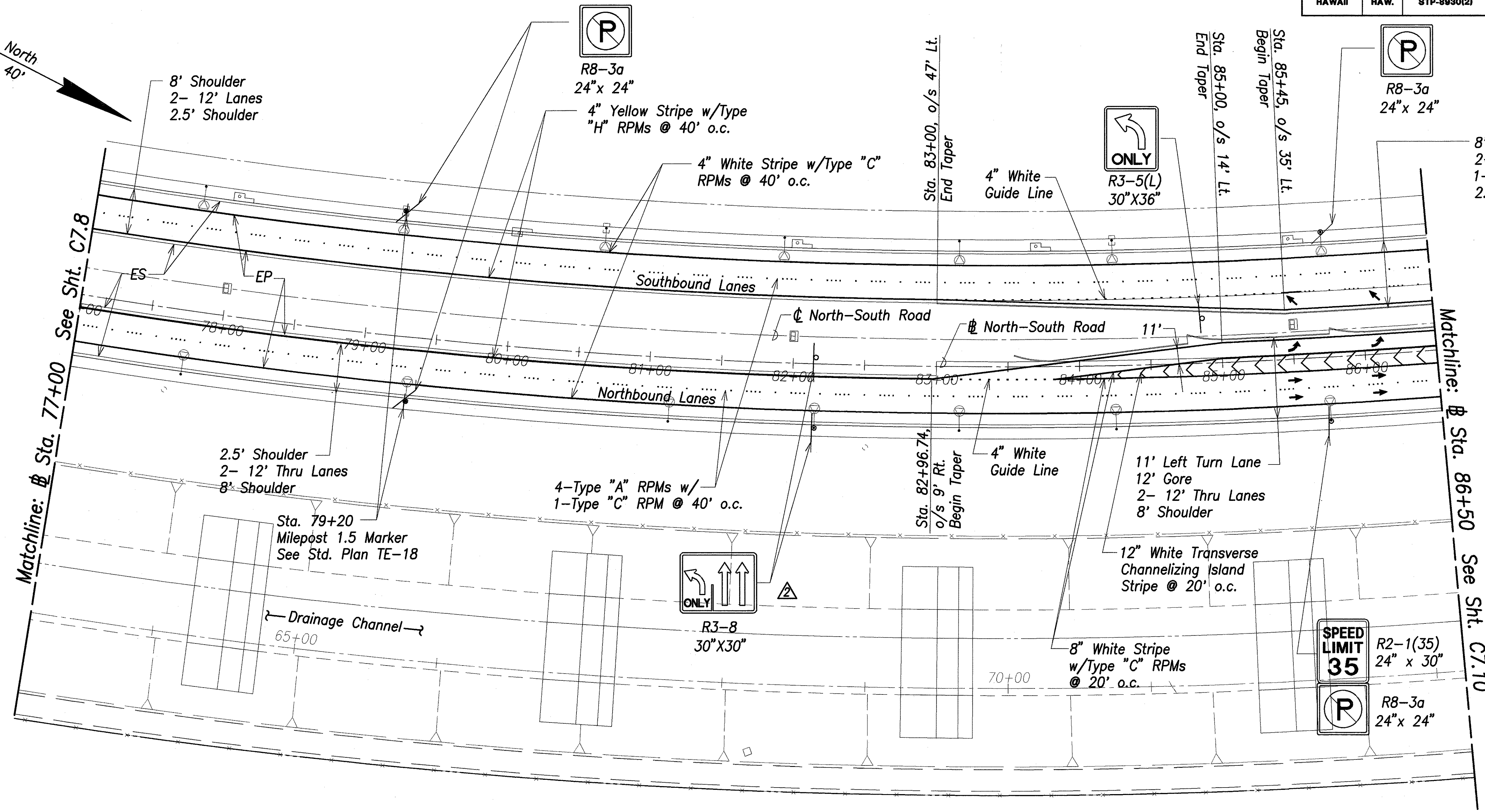
Striping Plan - Sta. 77+00 to Sta. 86+50 Scale: 1" = 40'
