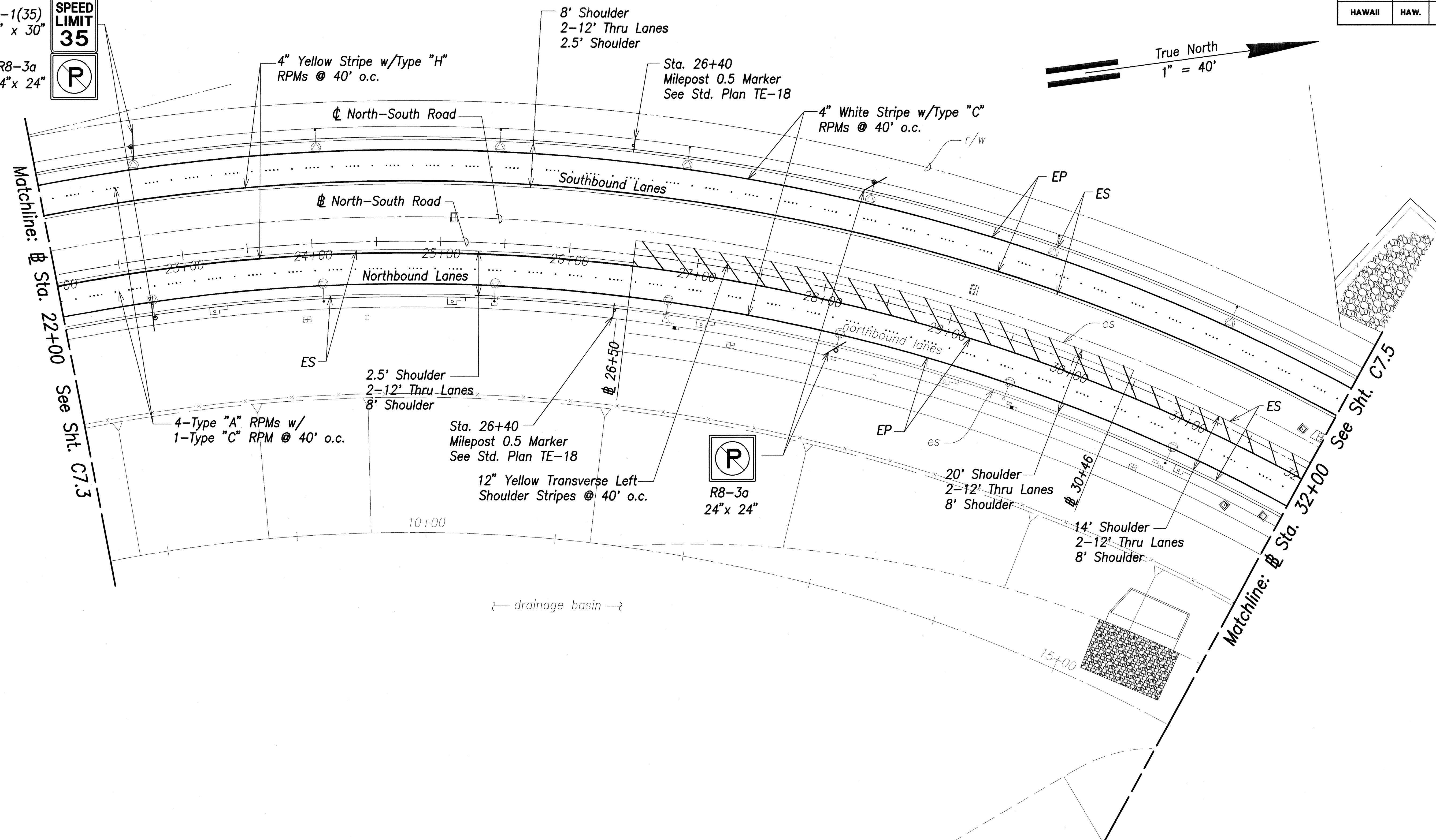
Striping Plan - Sta. 22+00 to Sta. 32+00 Scale: 1" = 40'
