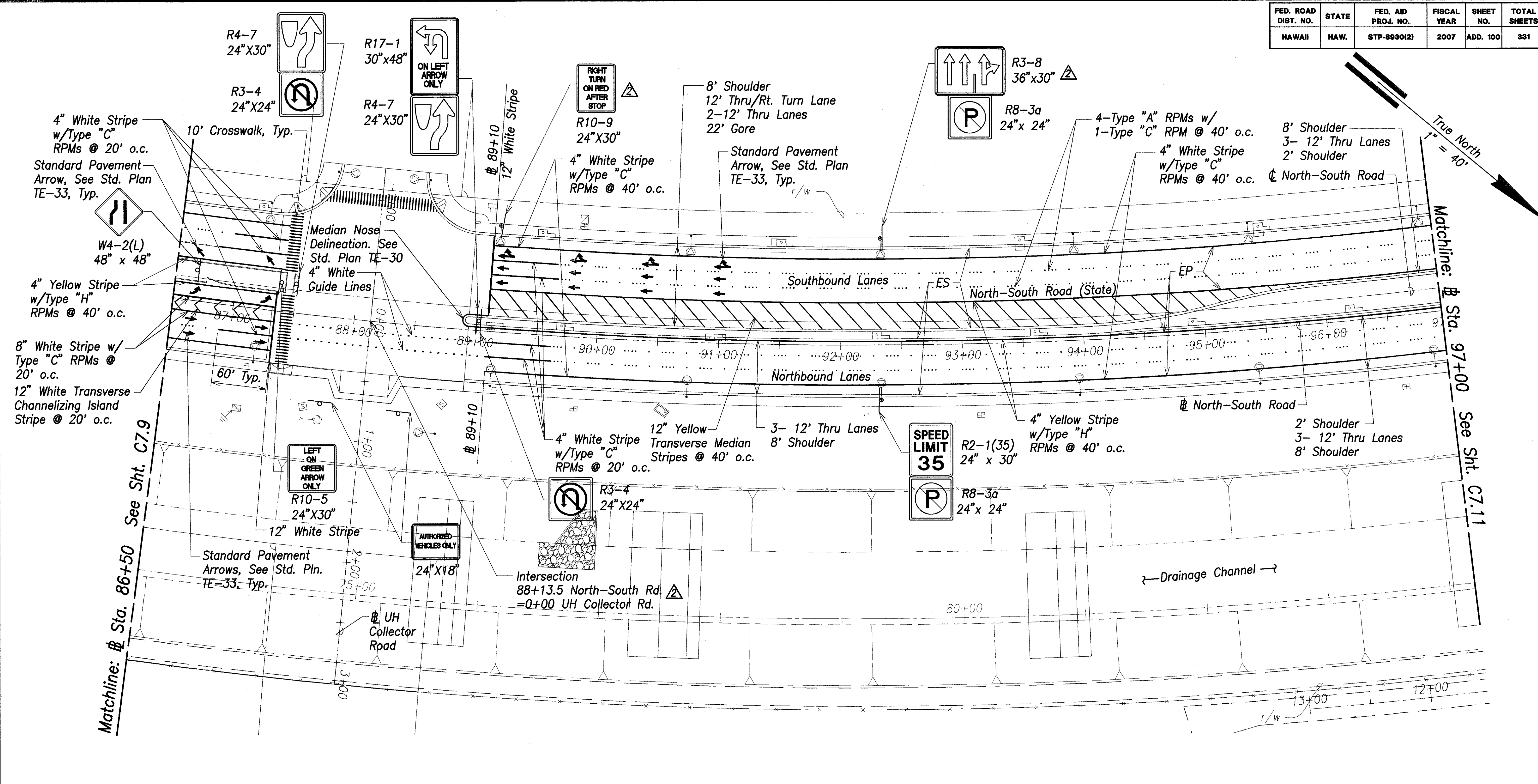
Striping Plan - Sta. 86+50 to Sta. 97+00 Scale: 1" = 40'
