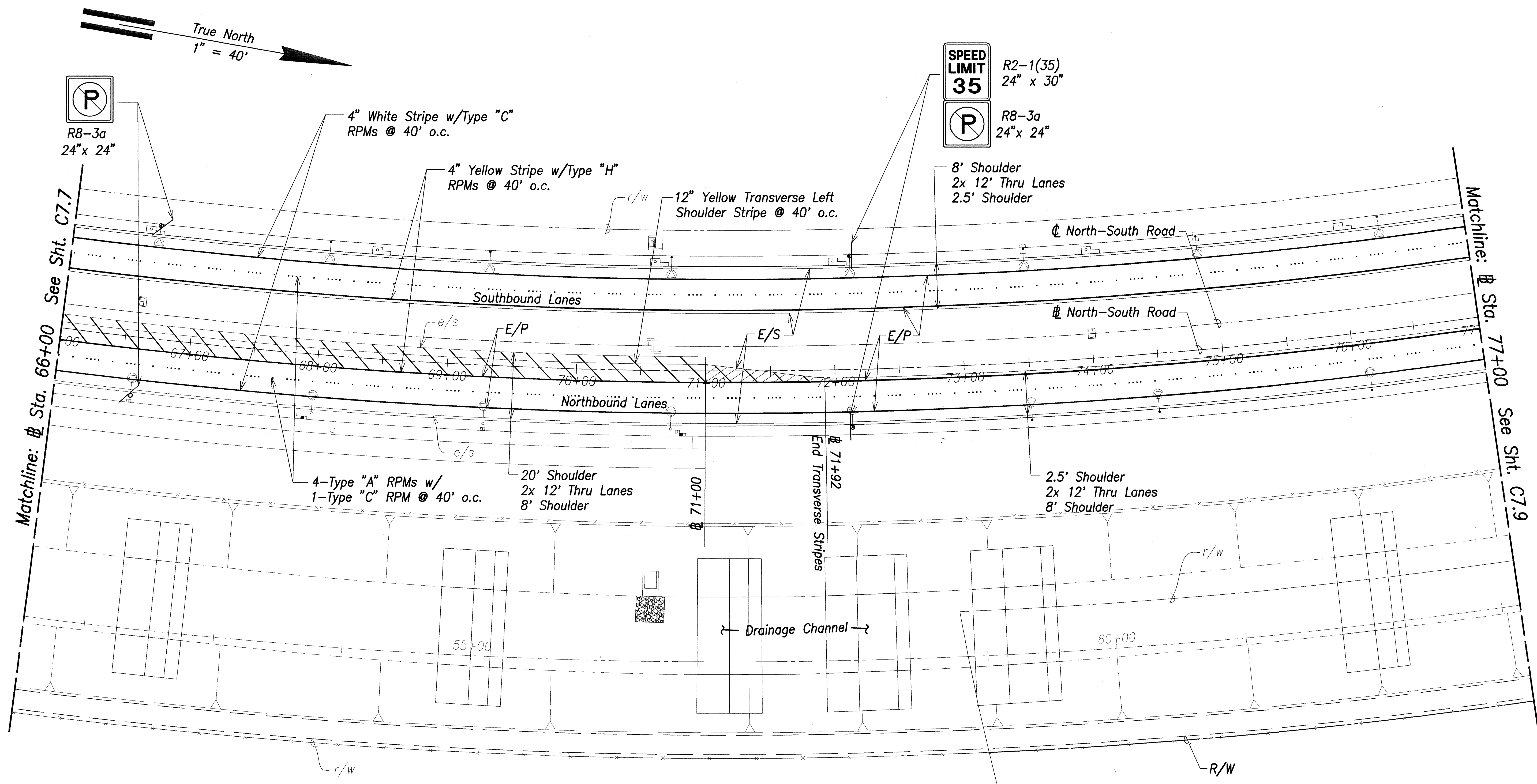
Striping Plan - Sta. 66+00 to Sta. 77+00 Scale: 1" = 40'
