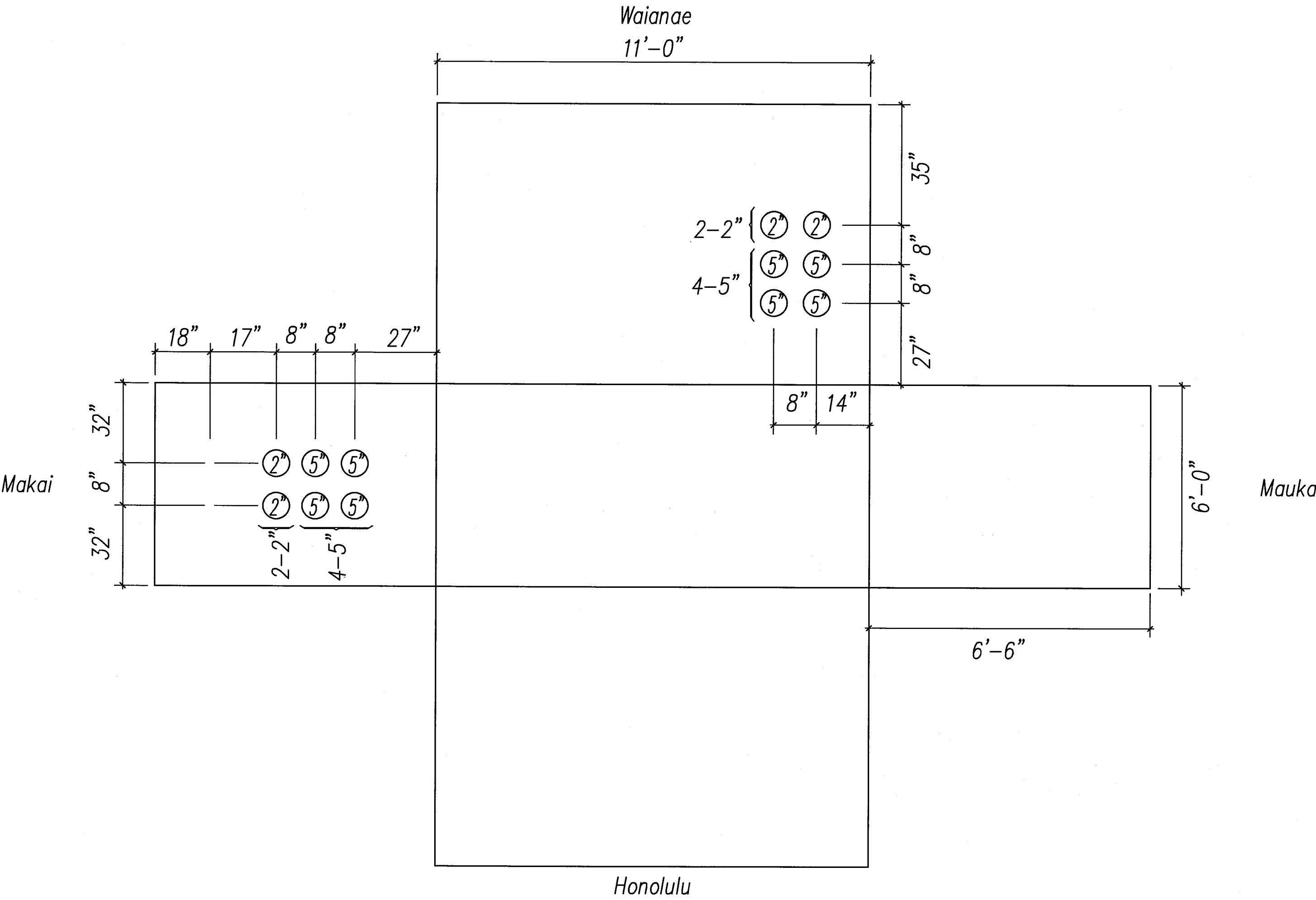
HECO 6' X 11' MANHOLE "F"
