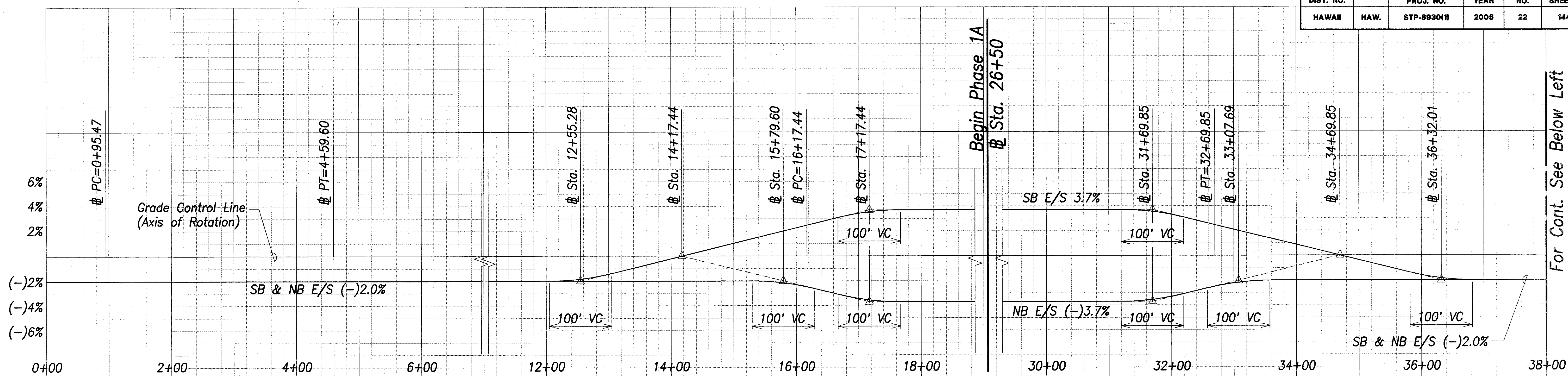
Superelevation Diagram, Sta. 0+00 - Sta. 38+00
