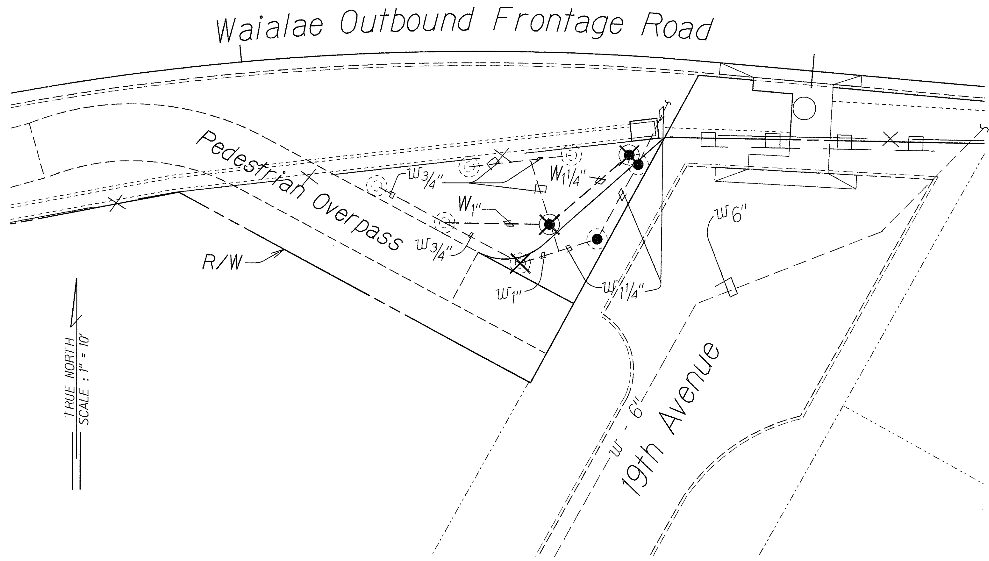
Plan Scale: 1" = 1.0'
