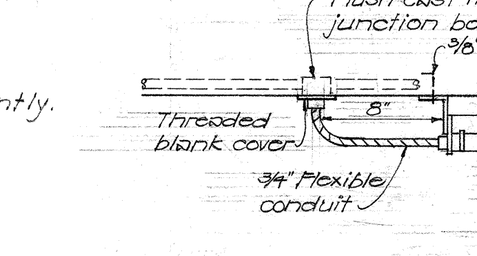
LONGITUDINAL SECTION Scale: 1"=10'
