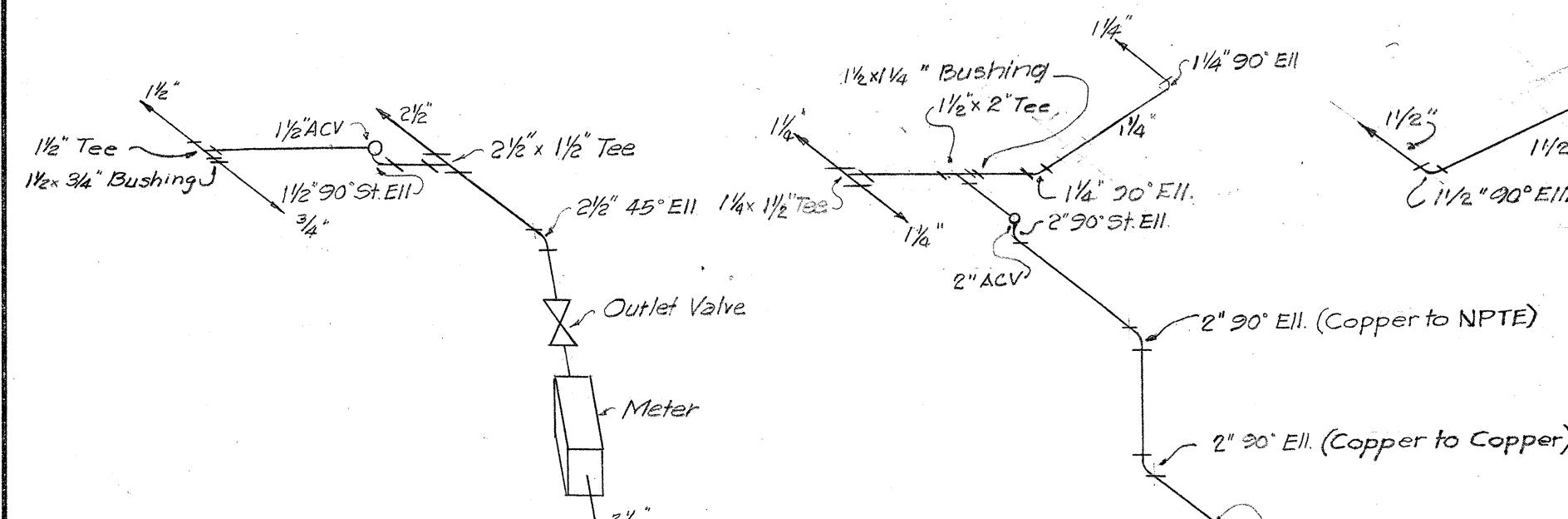
DETAIL 2-A
