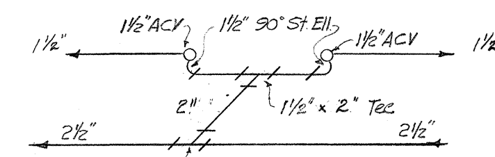
DETAIL 1-E
