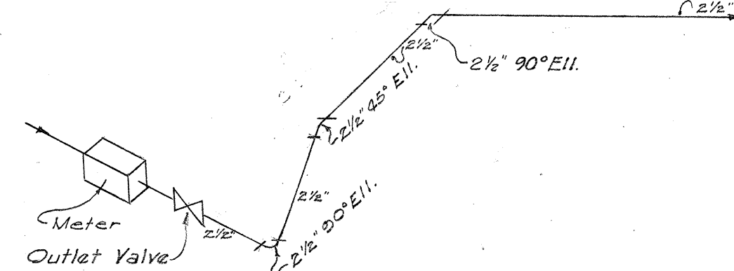
DETAIL 3-E
