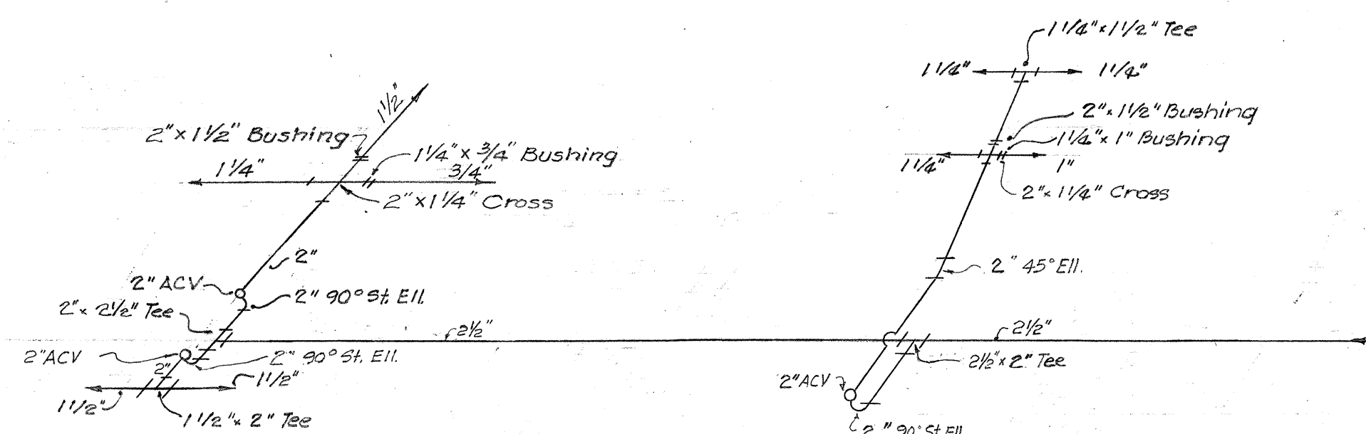
DETAIL 1-A
