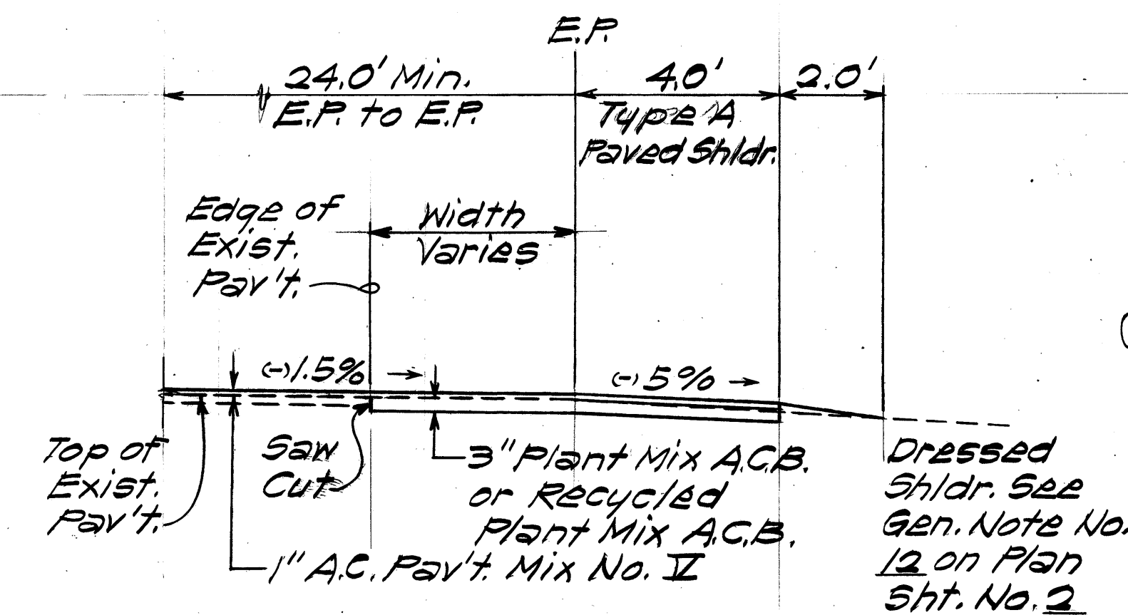
TYP. SECTION FOR PAY'T. WIDENING # STA. 19+50 TO # STA. 35+00 Scale: 3/8" = 1'-0"
