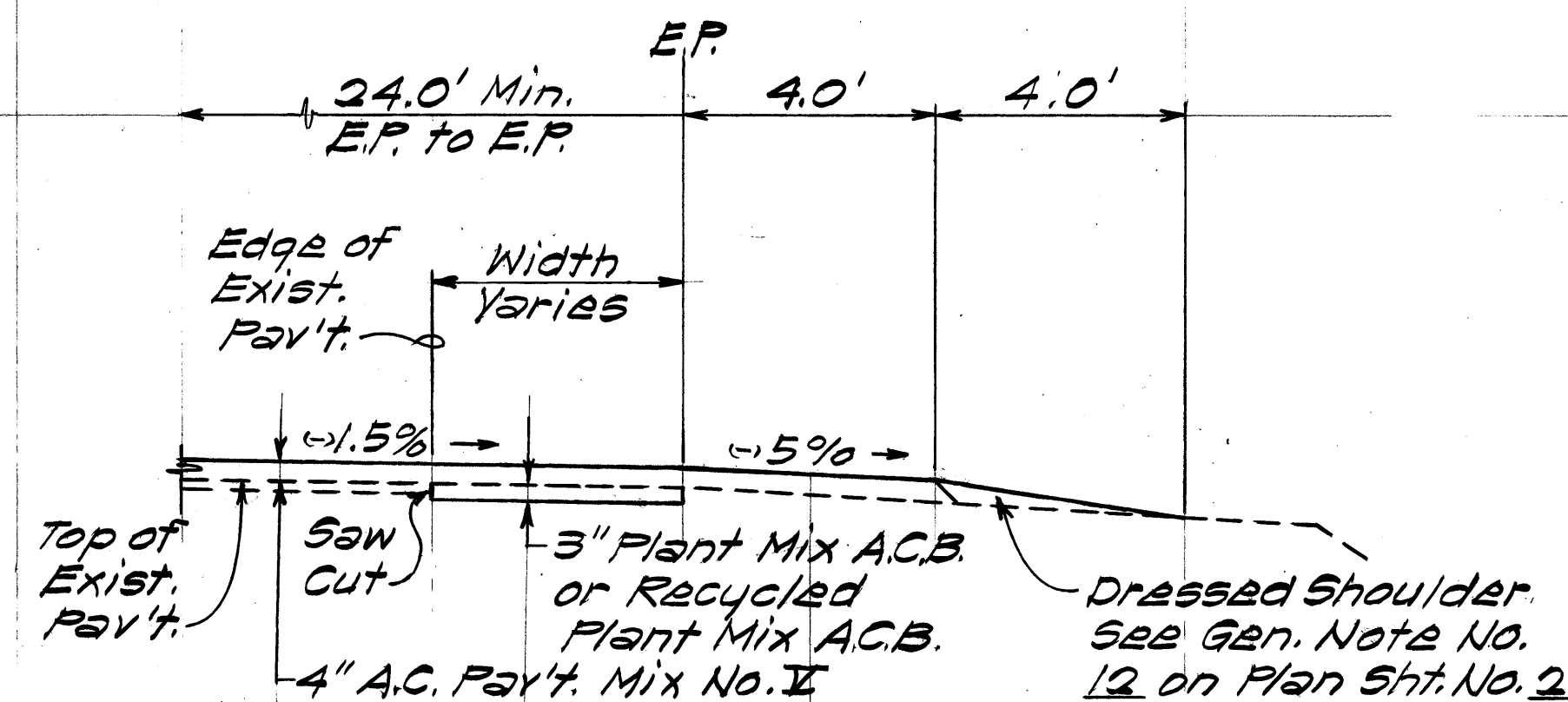
TYP. SECTION FOR PAY'T. WIDENING # STA. 5+00 TO # STA. 18+75 Scale: 3/8" = 1'-0"
