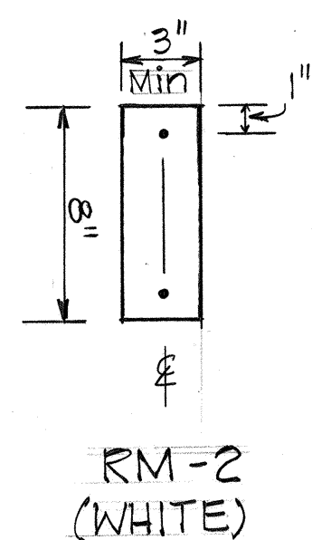
REFLECTOR MARKER N.T.S.
