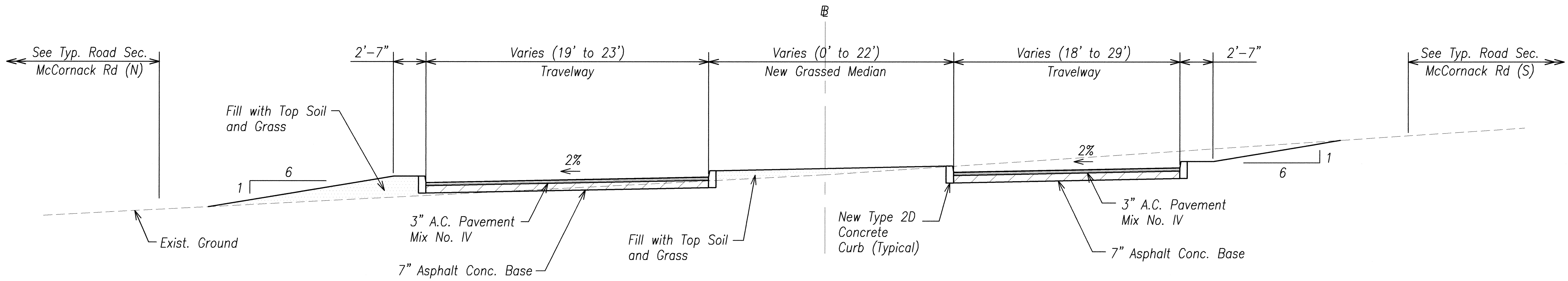
MC CORNACK RD (CENTER EXT.) @ STA. 22+39.37 to @ STA. 25+71.32 Scale: 1/4" = 1'-0"
