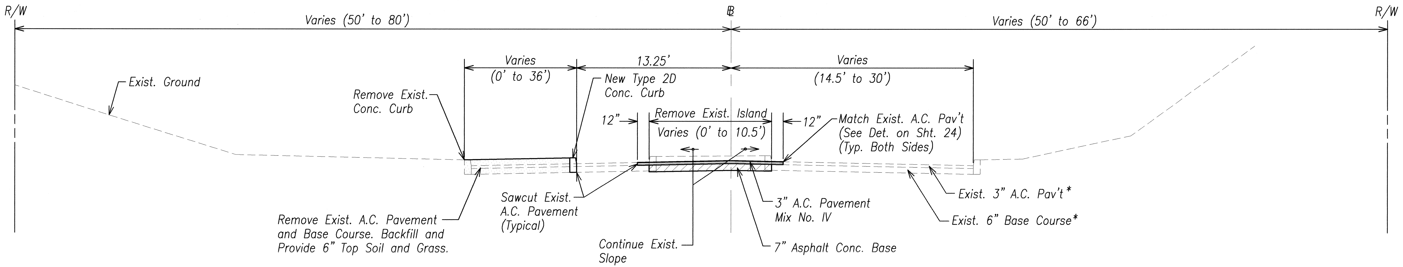
MC CORNACK RD (CENTER EXT.) @ STA. 22+31.46 to @ STA. 23+39.37 Scale: 1/4" = 1'-0"
