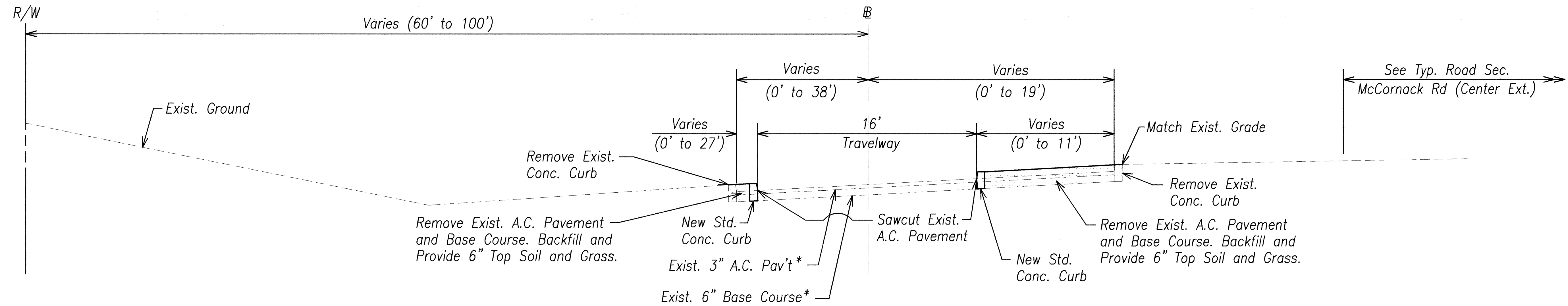
MC CORNACK RD (N) \pm STA. 23+35.56 to \pm STA. 27+89.06 Scale: 1/4" = 1'-0"
