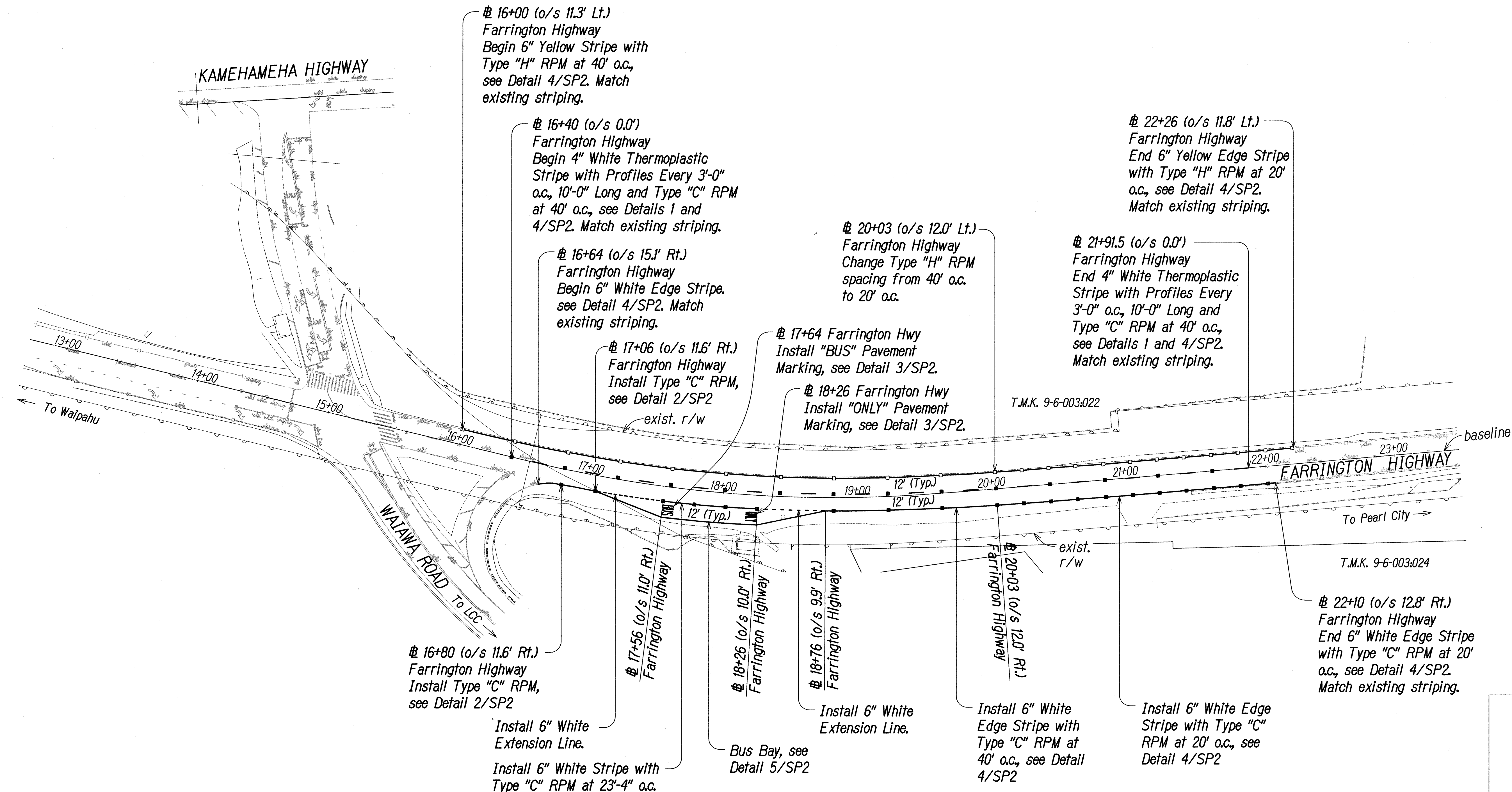
STRIPING PLAN Scale: 1" = 40'
