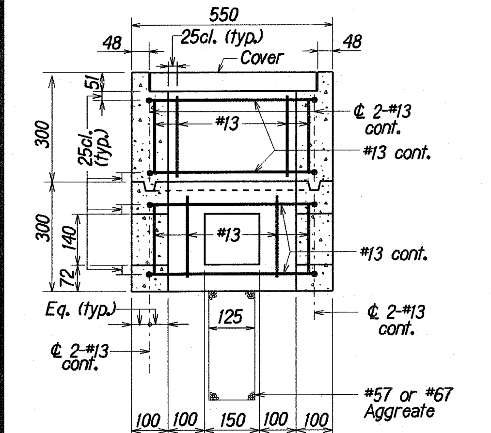
TYPE "A" PULLBOX (Old Type "B") Scale: 1 : 100
