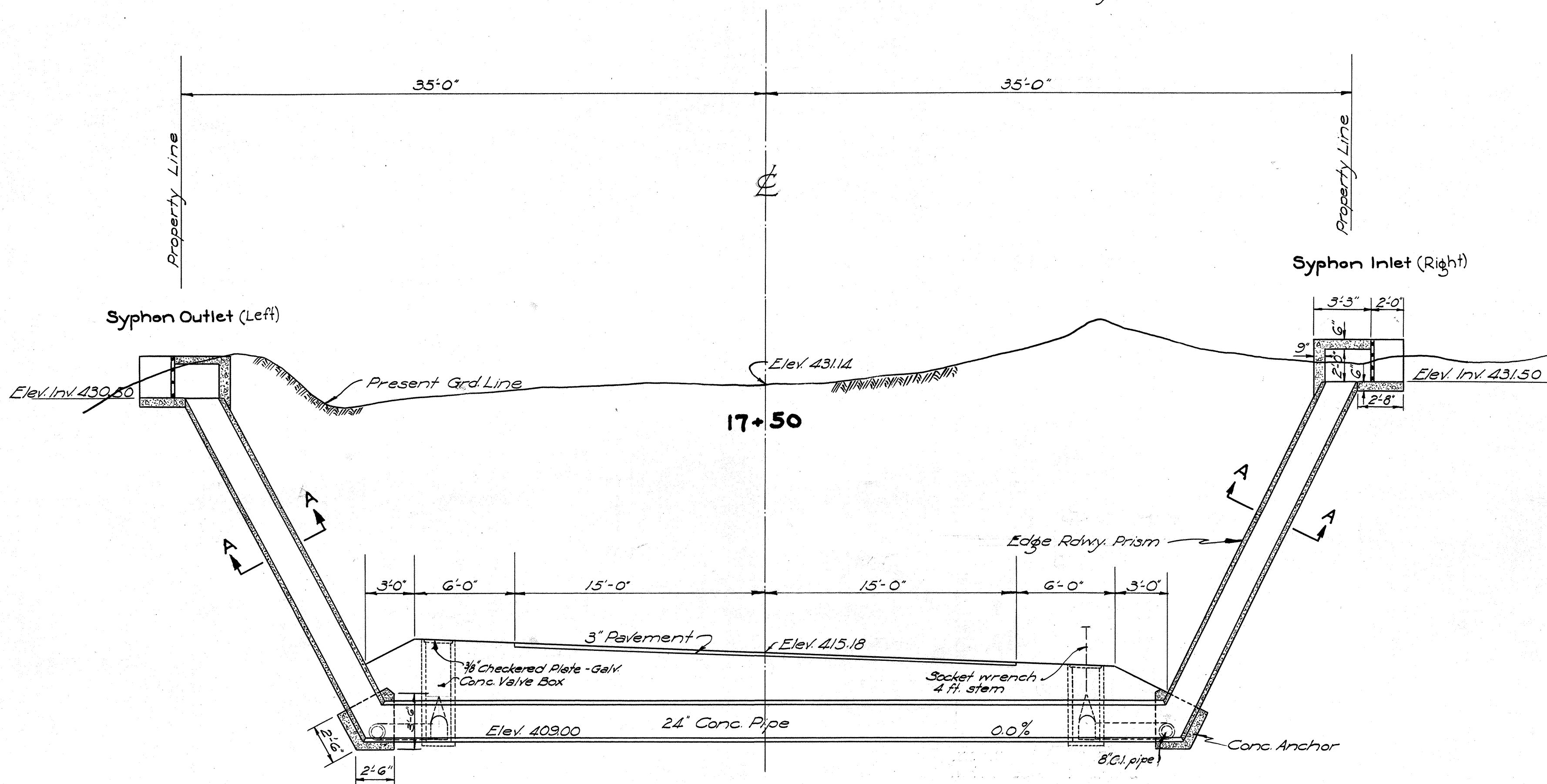
LONGITUDINAL SECTION 24" SYPHON Scale: 1"=5'-0"
