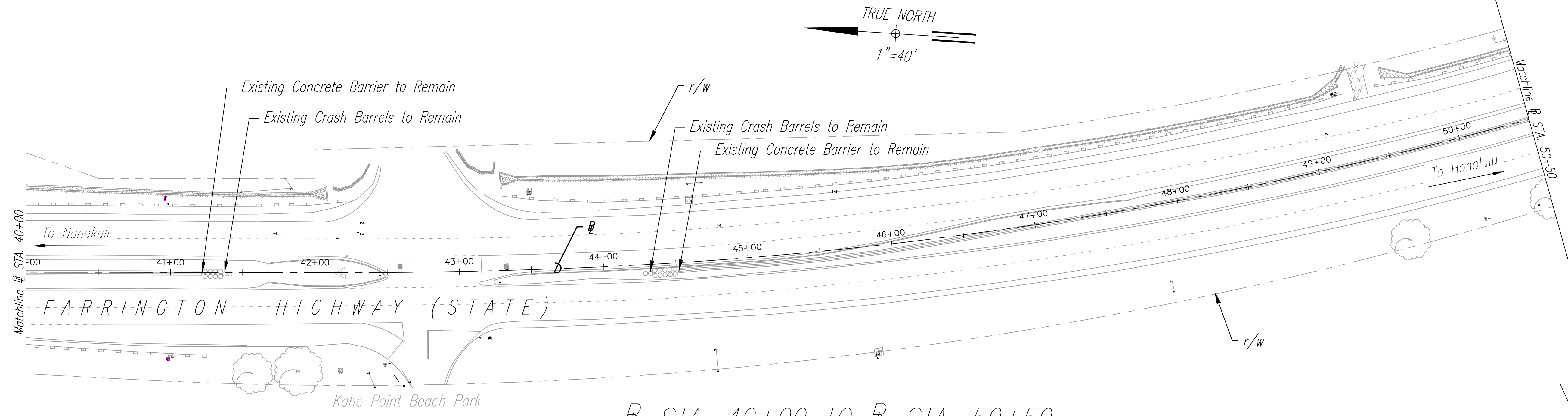
⌘ STA. 40+00 TO ⌘ STA. 50+50 Scale: 1" = 40'
