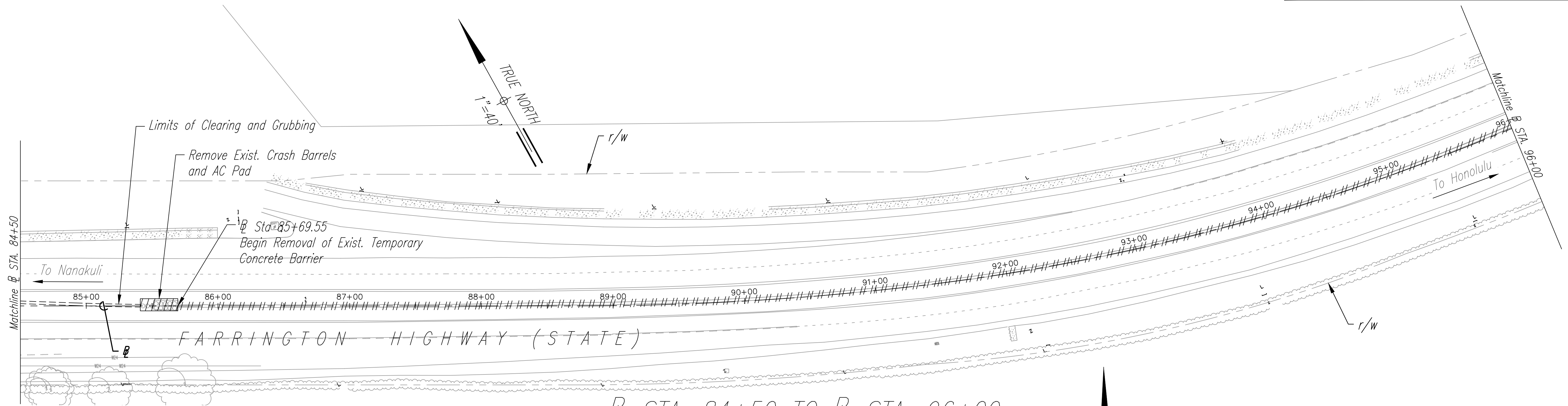
STA. 84+50 TO STA. 96+00 Scale: 1" = 40'
