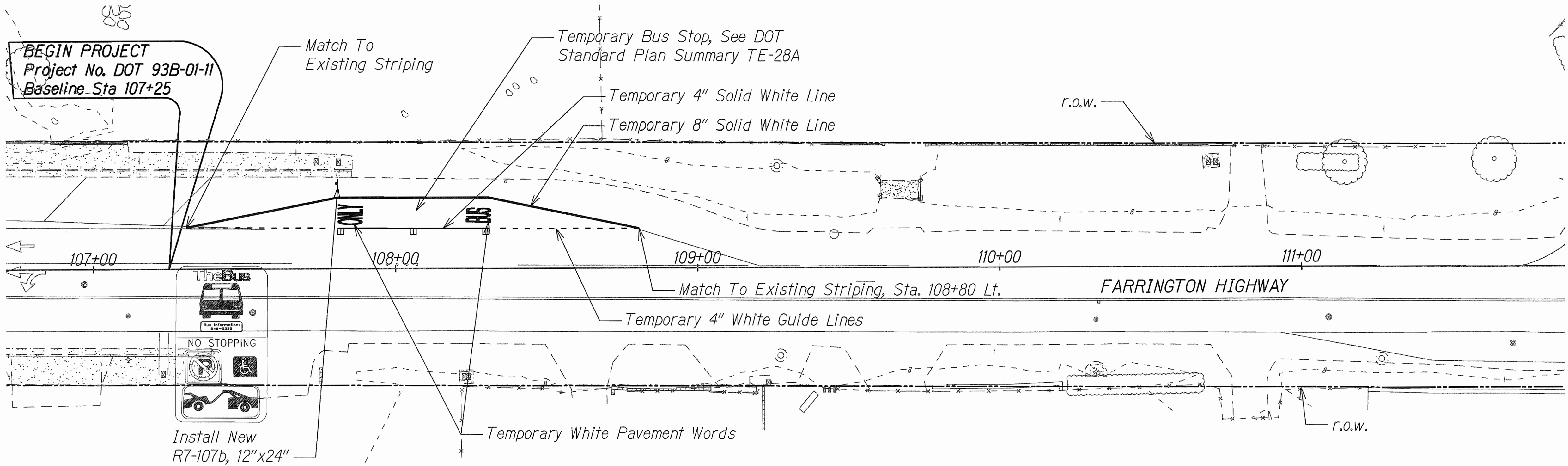
Demo Plan SCALE: 1" = 20'
