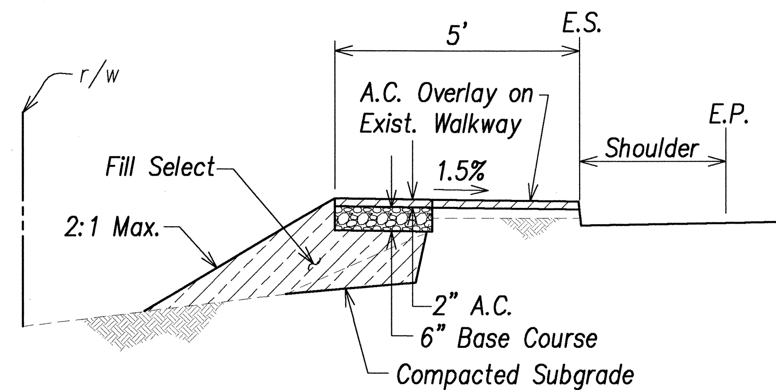
SECTION SCALE: 1" = 2' A 64 64
