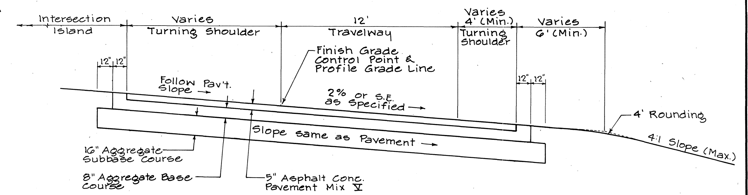
ROAD SECTION Access Road "Ba" Sta. 10+00 to Road "B" Sta. 1+58 Access Road "Bb" Sta. 10+00 to Sta. 12+86 Scale: 1" = 4'
