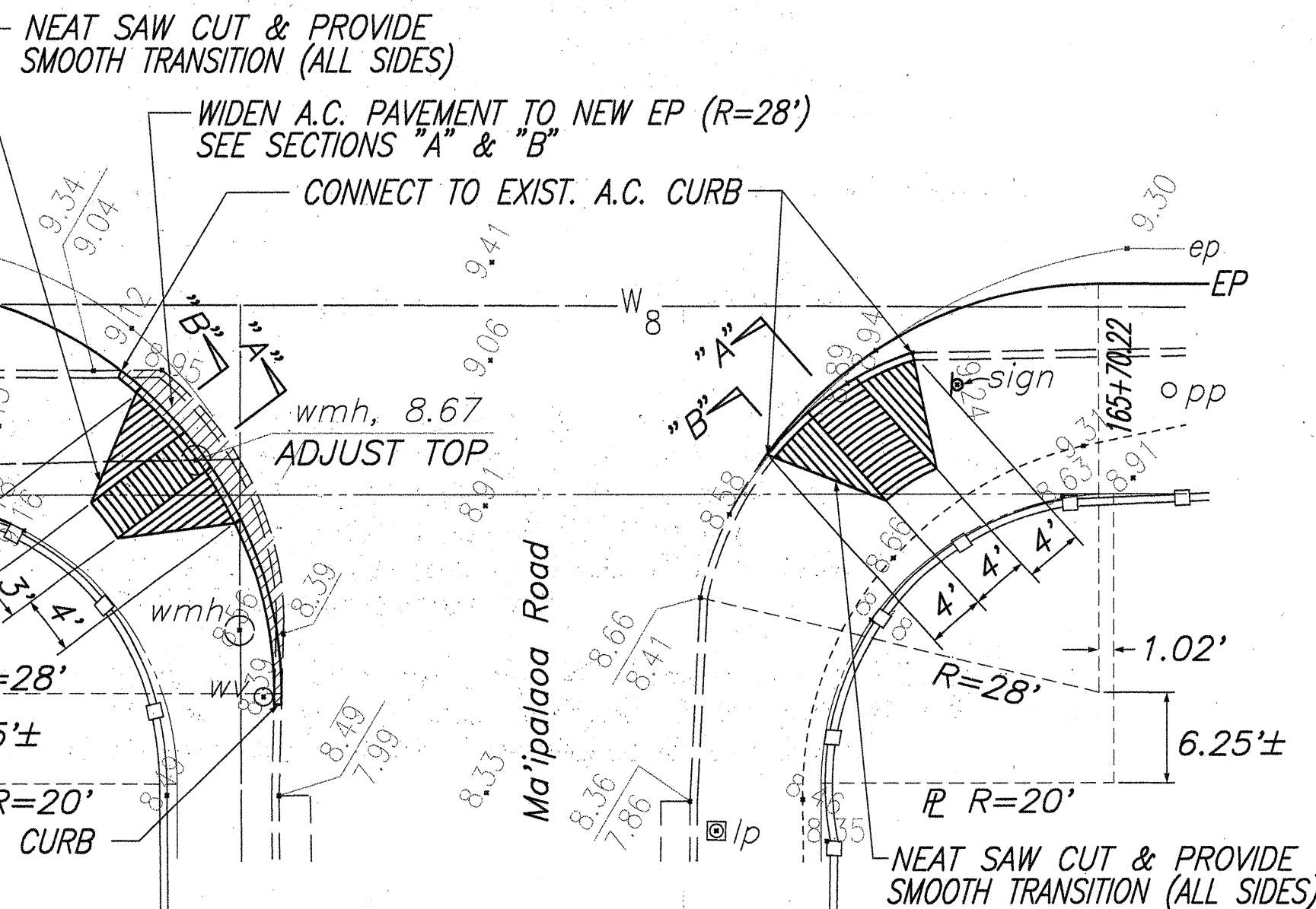
PLAN - A.C. RAMPS SCALE: 1" = 10'
