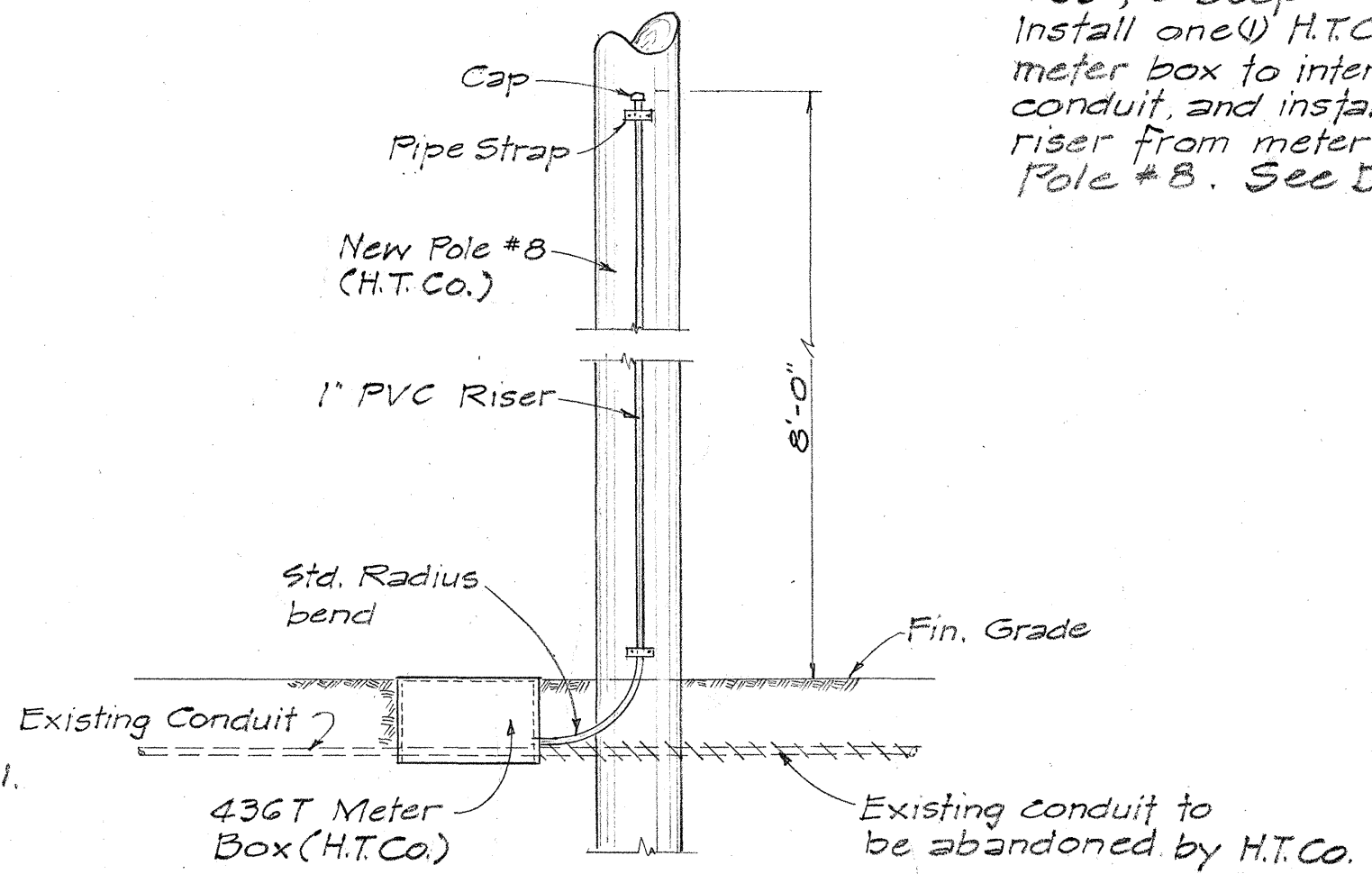
DETAIL AT POLE #8 (H.T.Co.)
