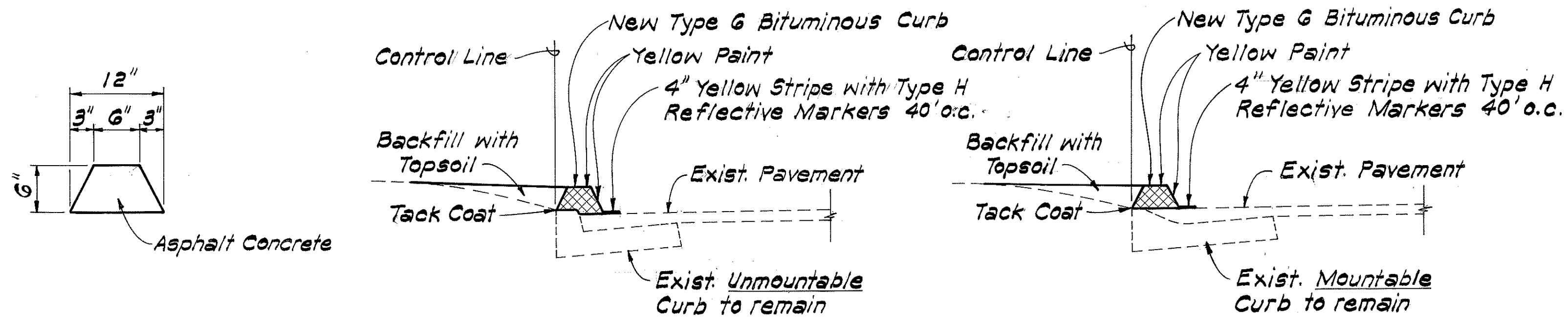
TYPE G BITUMINOUS CURB Scale: 1" = 1'-0"
