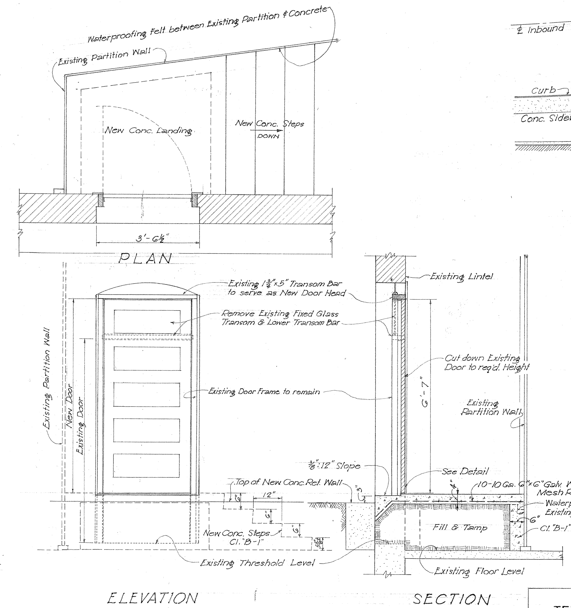
DOOR "B" Scale: 1/2" = 1'-0"
