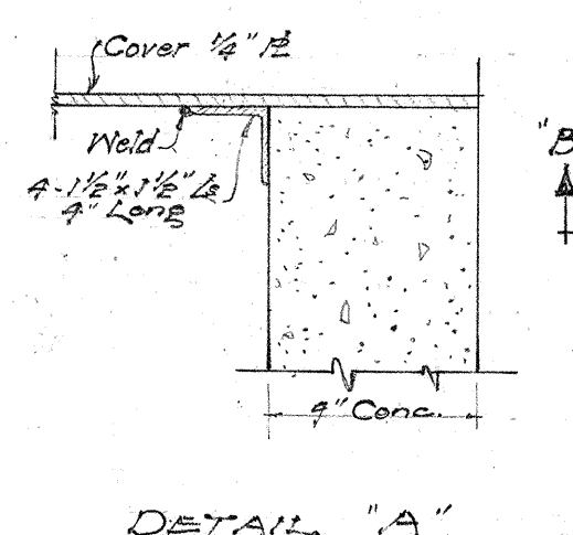
DETAIL "A" Scale: 1/2" = 1'-0"
