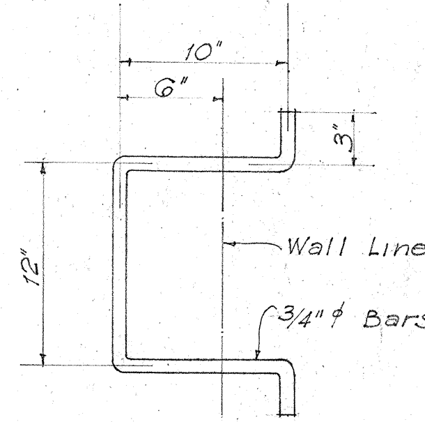
RUNG
