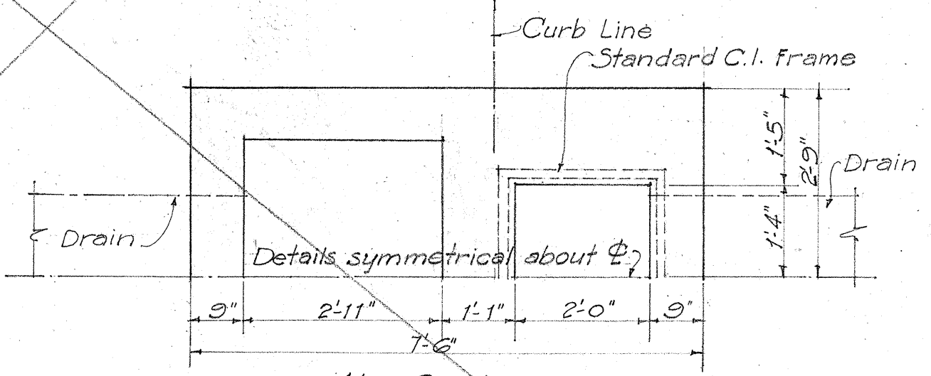
1/2 PLAN
