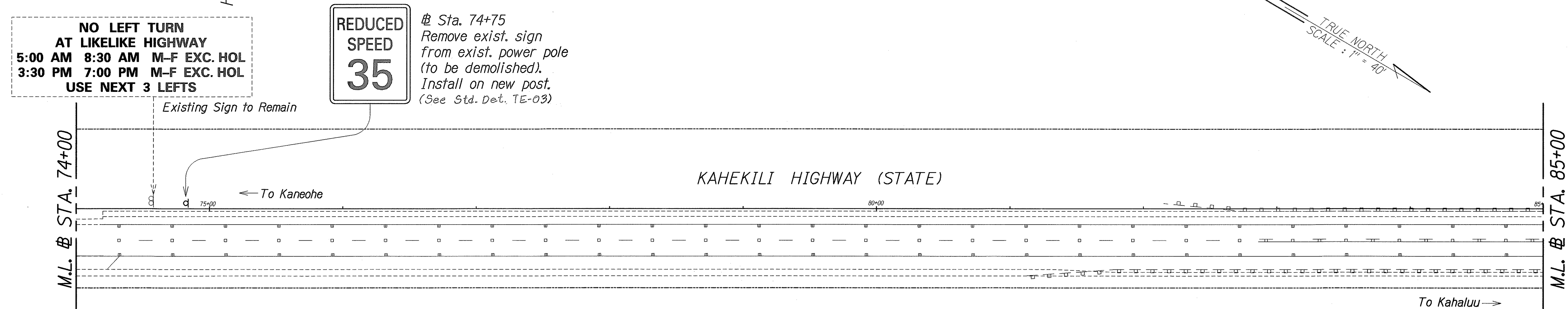
PLAN Scale: 1" = 40'
