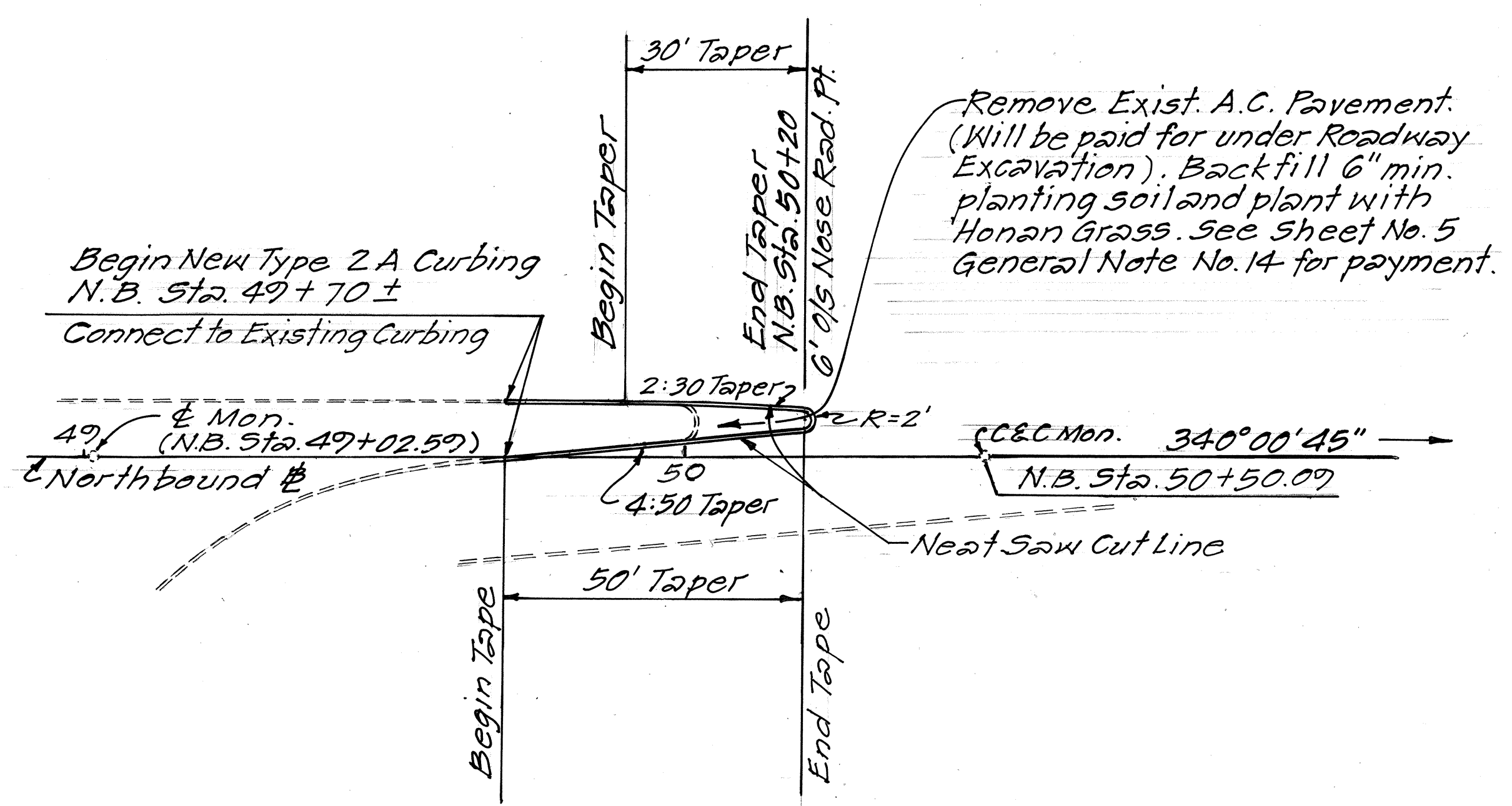
ISLAND RECONSTRUCTION DETAIL N.B. Sta. 49+70± to N.B. Sta. 50+22± Scale: 1" = 20'
