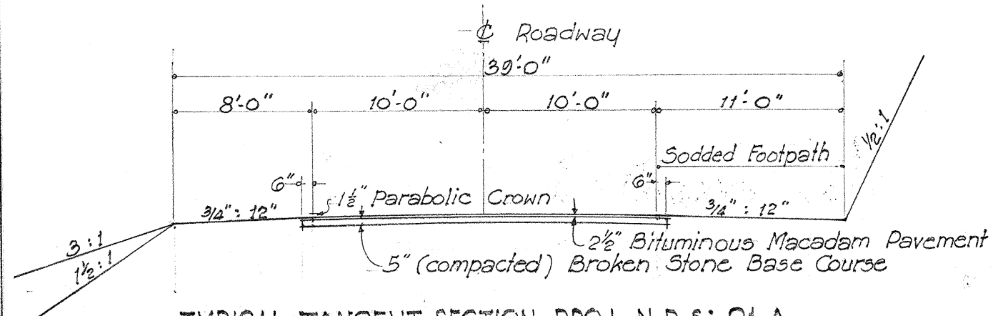
TYPICAL TANGENT SECTION-PROJ. N.R.S. 21 A
