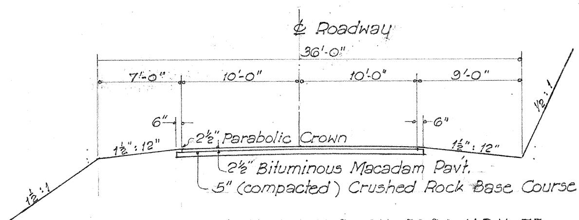
TYPICAL TANGENT SECTION - PROJ. N.R.H. 7E
