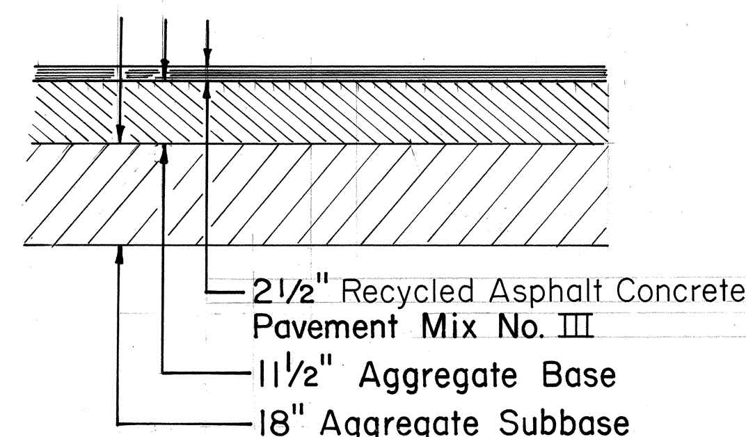
SECTION B Scale: 1/2" = 1' - 0"
