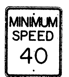
R2-4(40) 24"x 30" R2-4(40)-E 36"x 48" R2-4(40)-I 48"x 60"
