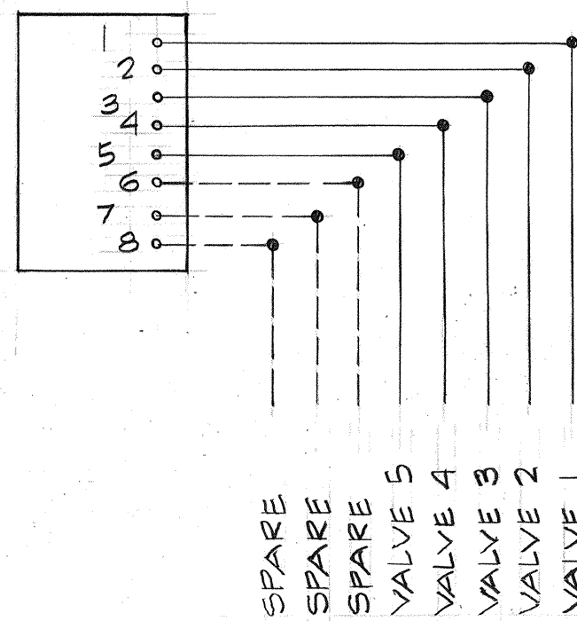
CONTROLLER "B" STA. 131+95
