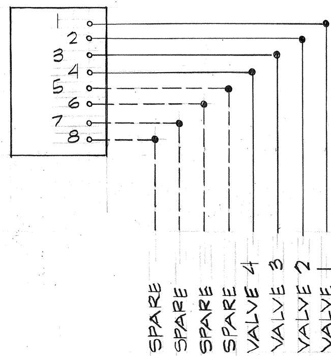
CONTROLLER "C" STA. 132+23
